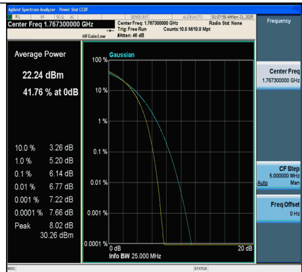
CA_66C-20MHz-10MHz-QPSK-QPSK-132473-132617-100RB#0-50RB#0-PASS
