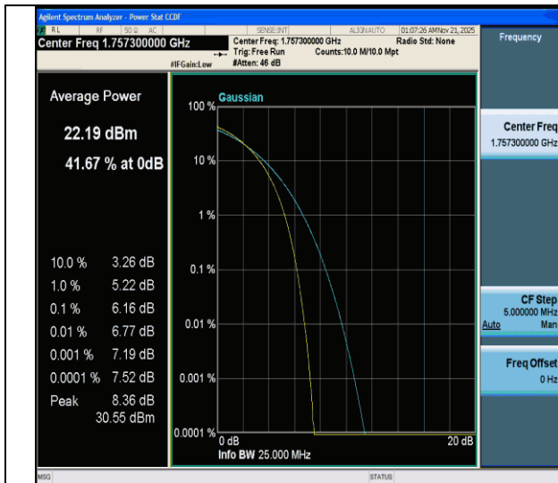
CA_66C-20MHz-10MHz-QPSK-QPSK-132373-132517-100RB#0-50RB#0-PASS
