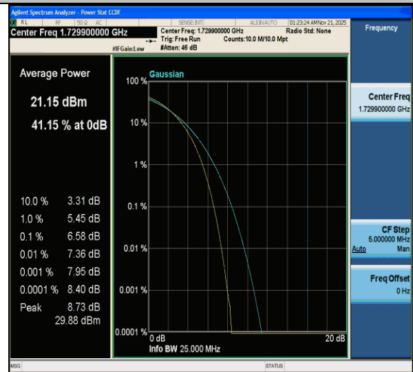
CA_66C-20MHz-20MHz-QPSK-QPSK-132072-132270-100RB#0-100RB#0-PASS
