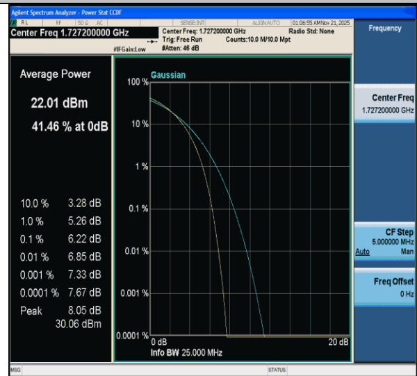
CA_66C-20MHz-10MHz-QPSK-QPSK-132072-132216-100RB#0-50RB#0-PASS
