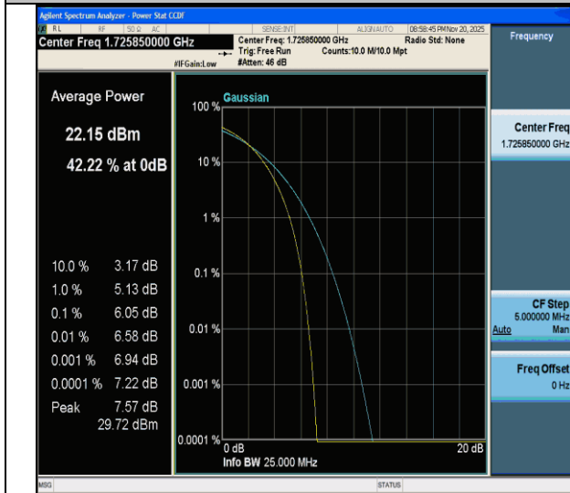
CA_66C-20MHz-5MHz-QPSK-QPSK-132072-132189-100RB#0-25RB#0-PASS
