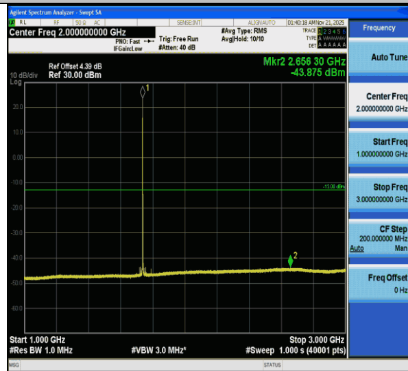
CA_66C-20MHz-20MHz-QPSK-QPSK-132323-132521-1RB#0- ORB#0-1000~3000MHz-PASS
