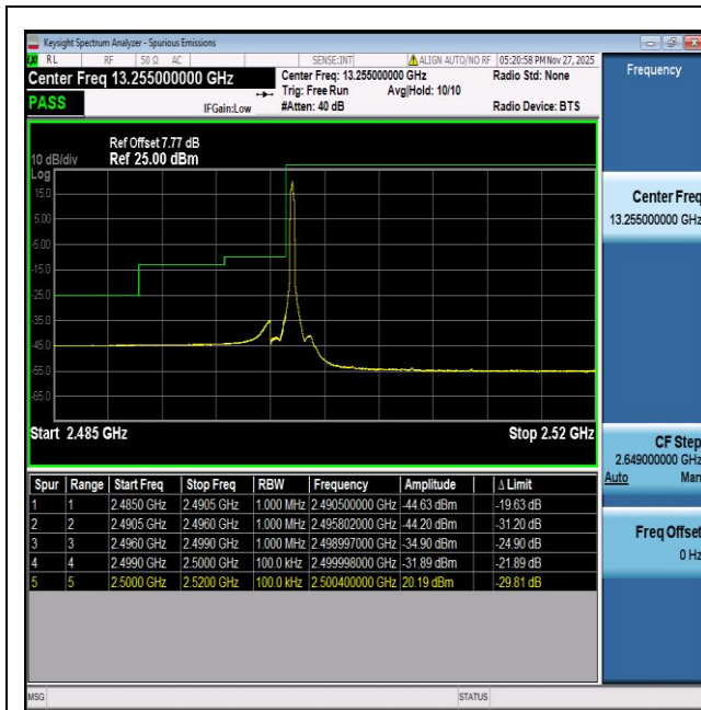
NTVN-n7-PC3-15-10-L-DFT-BPSK-Edge_1RB_Left-PASS
