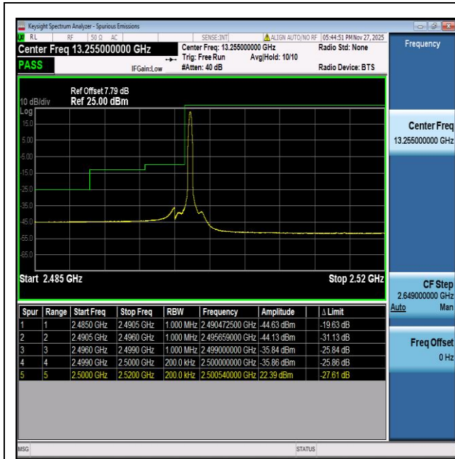
NTVN-n7-PC3-15-20-L-DFT-BPSK-Edge_1RB_Left-PASS
