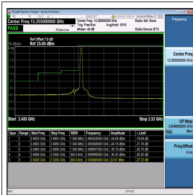
NTVN-n7-PC3-15-30-L-DFT-BPSK-Edge_1RB_Left-PASS
