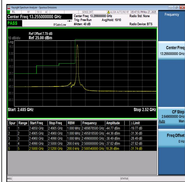
NTVN-n7-PC3-15-20-L-CP-QPSK-Edge_1RB_Left-PASS
