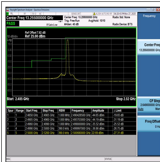
NTVN-n7-PC3-15-40-L-DFT-BPSK-Edge_1RB_Left-PASS
