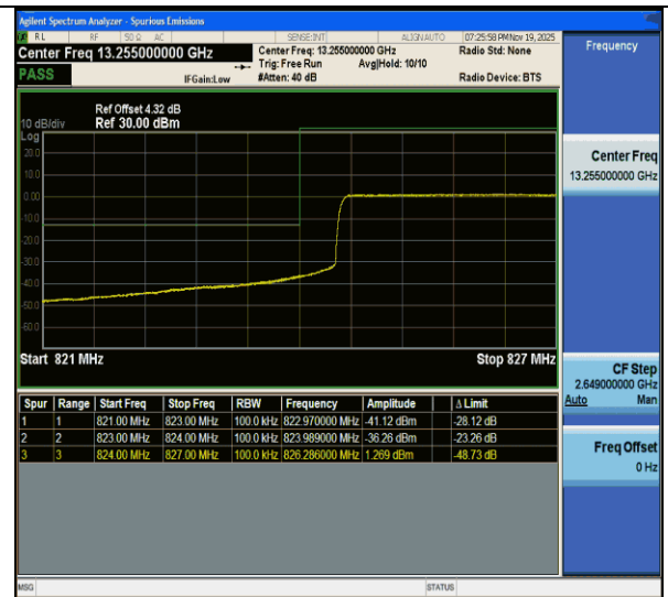
Band26(824-849)-10MHz-QPSK-26840-50RB#0-PASS
