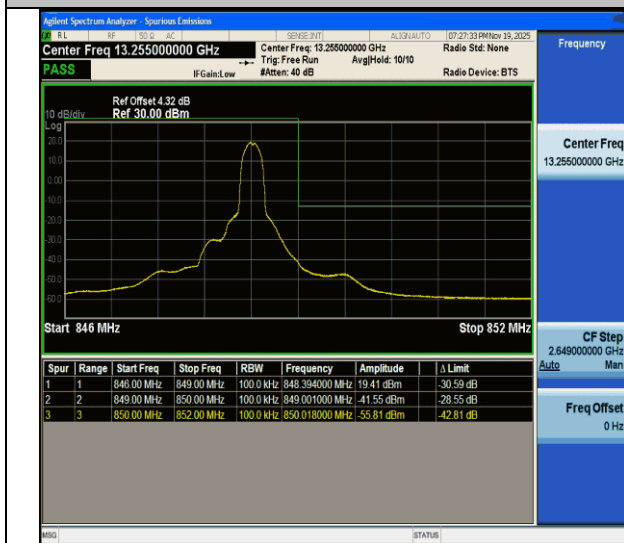
Band26(824-849)-10MHz-QPSK-26990-1RB#49-PASS
