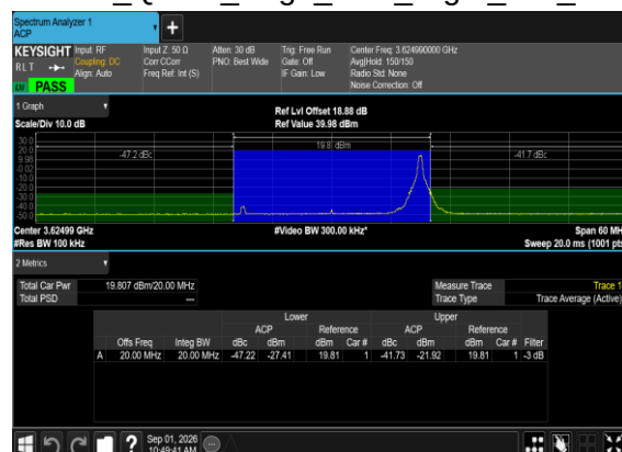
N48(20M)_DFT-s- OFDM QPSK Edge 1RB Right Mid CH
