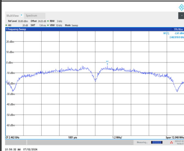
MIMO Ant 1
