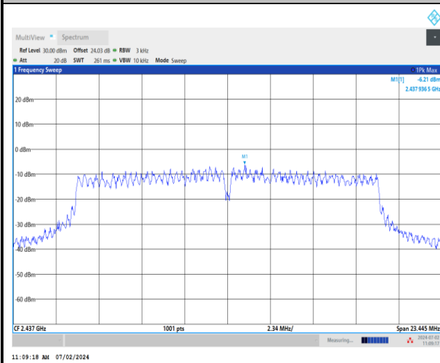
MIMO Ant 1
