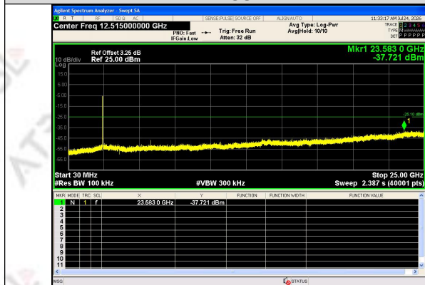
30.0 MHz - 25000.0 MHz IEEE 802.11ax_Channel 6_40MHz_Antenna 0_RU&Index SU
