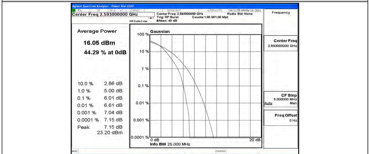
Band41-20MHz-16QAM-41490-1RB#0
