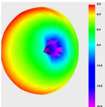
ANT2: 800Mhz
