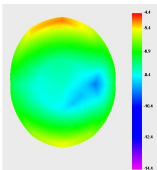
ANT2: 900Mhz
