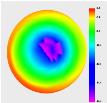
ANT1: 700Mhz
