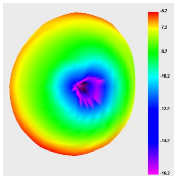
ANT2: 700Mhz
