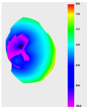
ANT2: 1900Mhz
