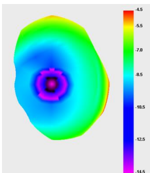
ANT2: 1700Mhz
