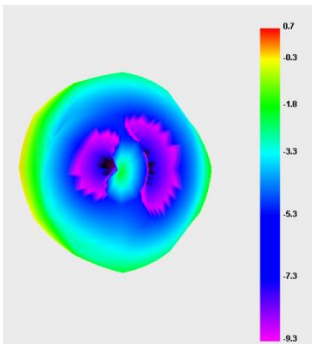
ANT1: 1700Mhz
