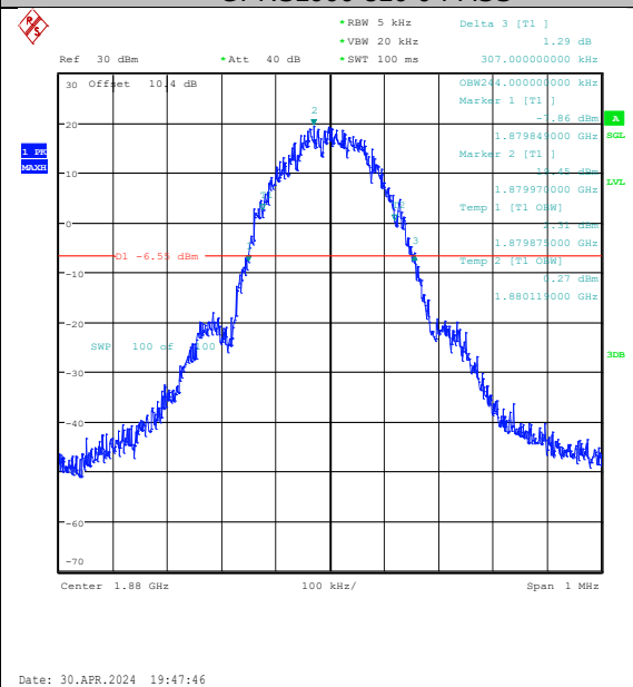
EGPRS1900-661-2-PASS
