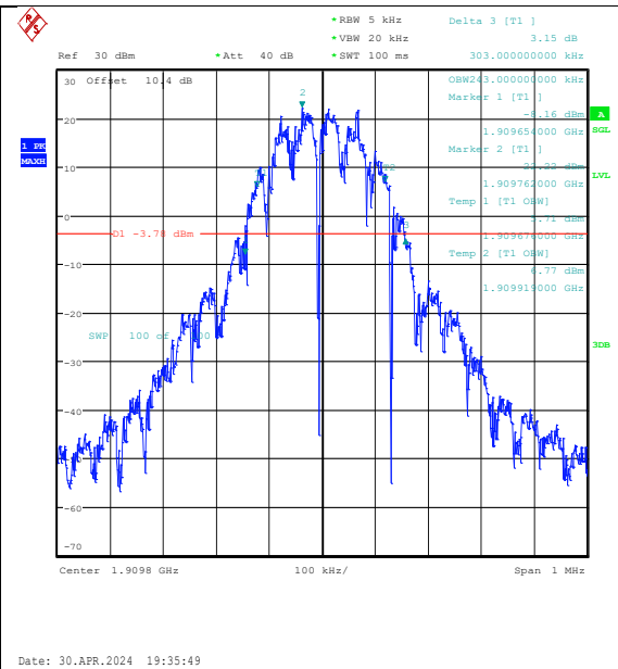
GPRS1900-810-0-PASS
