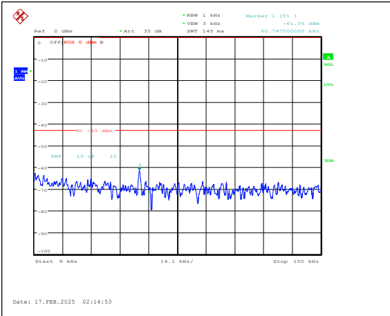
Band25-1.4MHz-QPSK-26365-1RB#0-0.009~0.15 -PASS
