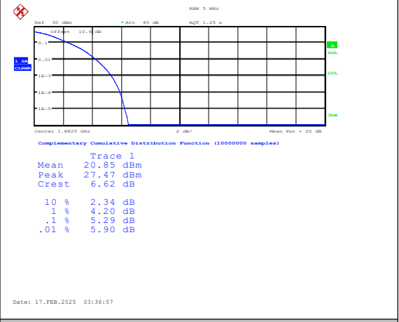
Band25-5MHz-QPSK-26365-25RB#0-PASS
