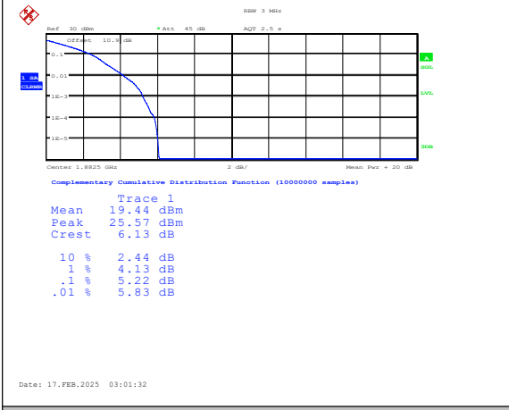
Band25-3MHz-QPSK-26365-1RB#0-PASS
