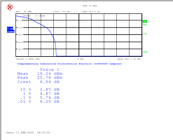
Band25-10MHz-16QAM-26365-1RB#0-PASS
