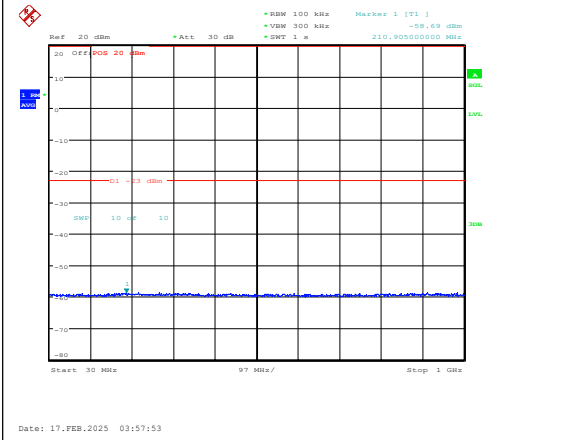
Band25-10MHz-QPSK-26365-1RB#0-30~1000-P ASS
