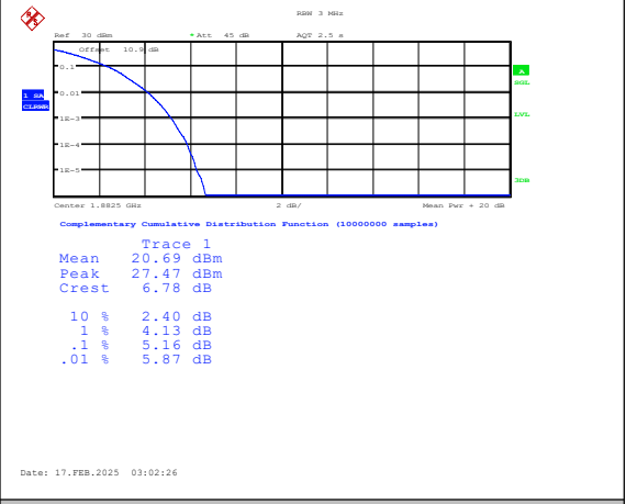
Band25-3MHz-QPSK-26365-15RB#0-PASS
