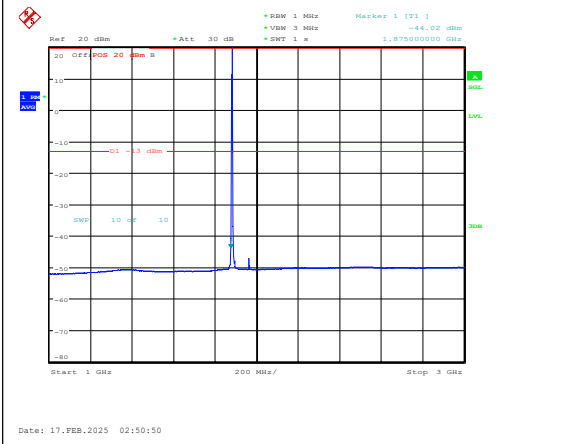
Band25-3MHz-16QAM-26365-1RB#0-1000~3000 -PASS
