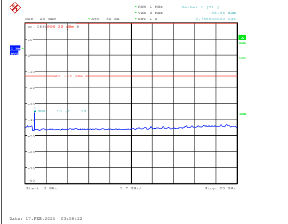
Band25-10MHz-QPSK-26365-1RB#0-3000~2000 0-PASS
