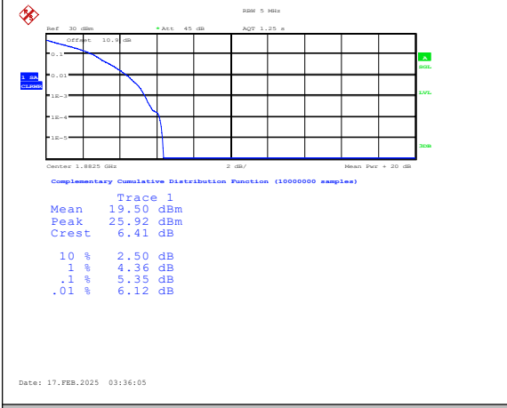
Band25-5MHz-QPSK-26365-1RB#0-PASS
