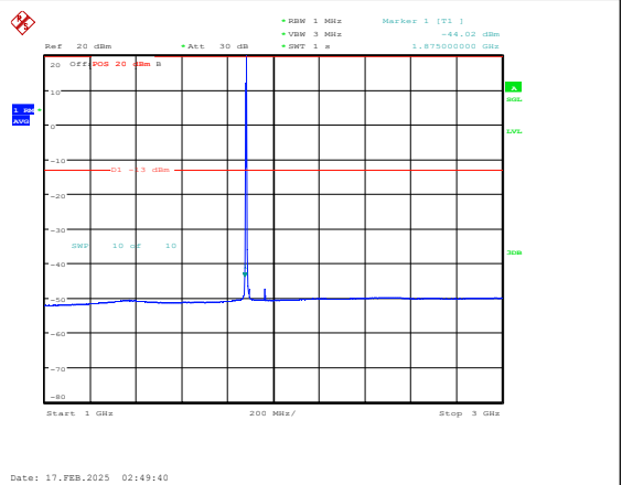
Band25-3MHz-QPSK-26365-1RB#0-1000~3000-P
