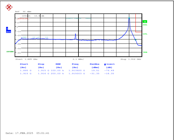
Band25-20MHz-QPSK-26590-1RB#99-PASS
