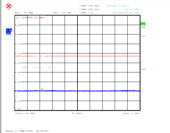
Band25-3MHz-QPSK-26365-1RB#0-30~1000-PA
