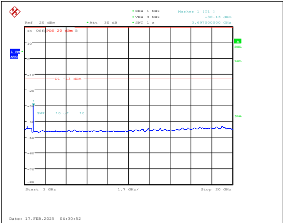
Band25-15MHz-QPSK-26115-1RB#0-3000~2000 0-PASS
