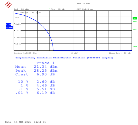
Band25-10MHz-QPSK-26365-50RB#0-PASS
