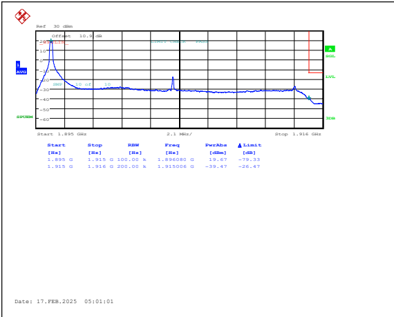
Band25-20MHz-QPSK-26590-1RB#0-PASS
