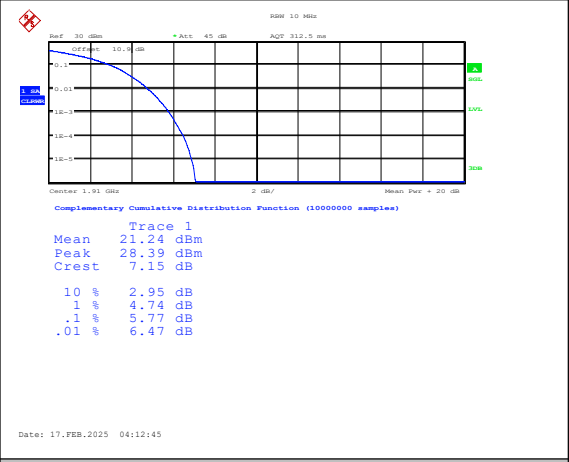
Band25-10MHz-QPSK-26640-50RB#0-PASS
