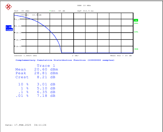
Band25-10MHz-16QAM-26365-50RB#0-PASS
