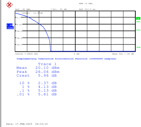
Band25-10MHz-QPSK-26365-1RB#0-PASS
