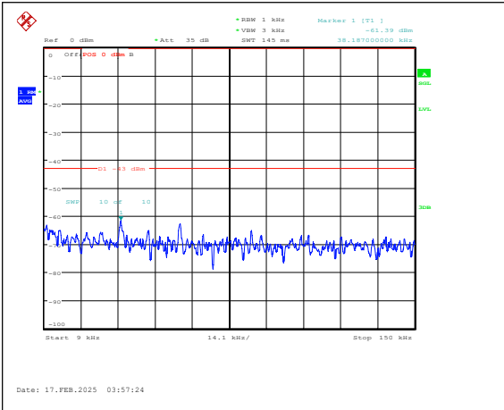
Band25-10MHz-QPSK-26365-1RB#0-0.009~0.15 -PASS
