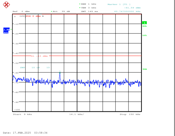
Band25-10MHz-16QAM-26365-1RB#0-0.009~0.15 -PASS
