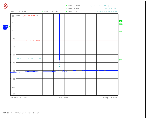
Band25-3MHz-QPSK-26675-1RB#0-1000~3000-P ASS
