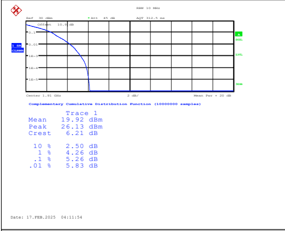
Band25-10MHz-QPSK-26640-1RB#0-PASS
