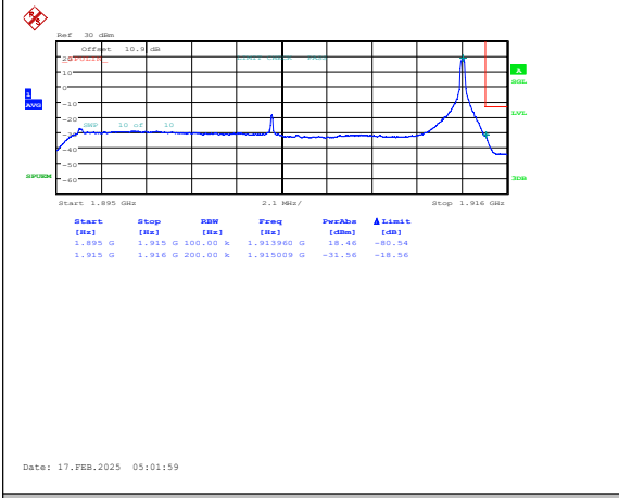
Band25-20MHz-16QAM-26590-1RB#99-PASS
