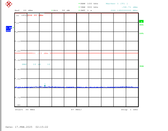
Band25-1.4MHz-QPSK-26365-1RB#0-30~1000-P ASS
