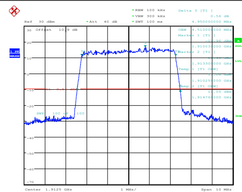
Band25-5MHz-QPSK-26365-25RB#0-PASS
