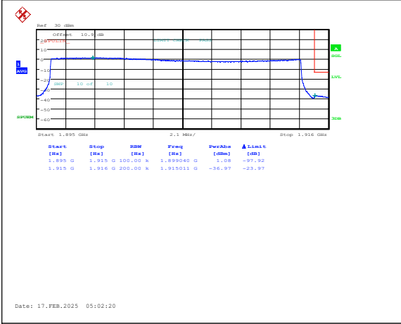
Band25-20MHz-QPSK-26590-100RB#0-PASS
