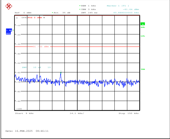
Band5-3MHz-QPSK-20635-1RB#0-0.009~0.15-PASS
