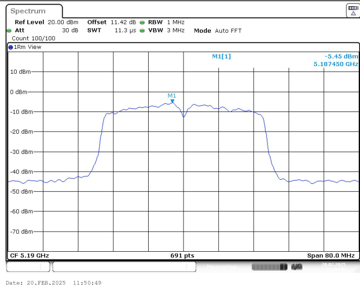
11AC40MIMO_Ant1_5190
