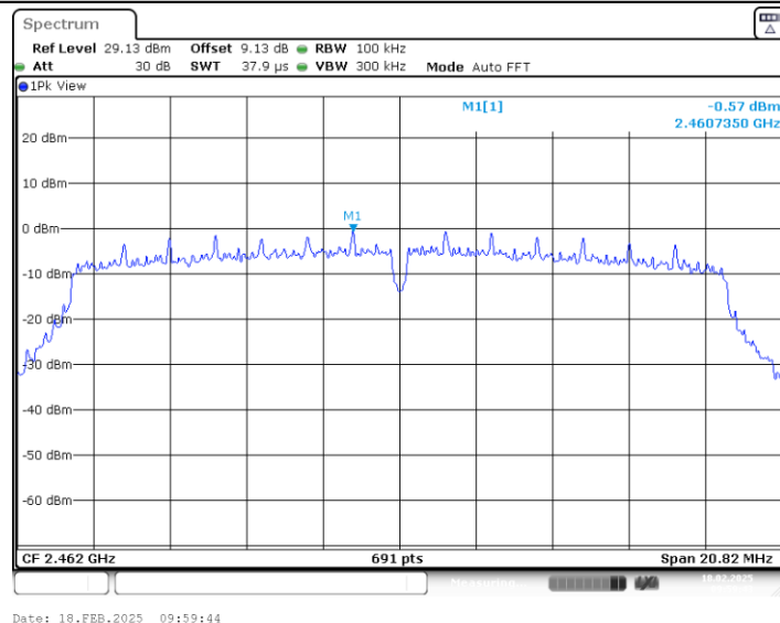
11N20MIMO_2462
