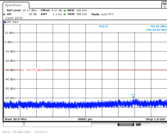
11G_Ant2_2412_30~1000
