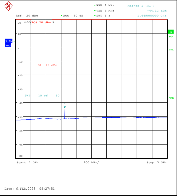
Band26(824-849)-1.4MHz-QPSK-26797-6RB#0-1 000~3000-PASS
