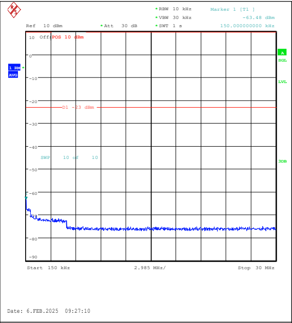
Band26(824-849)-1.4MHz-QPSK-26797-6RB#0-0. 15~30-PASS
