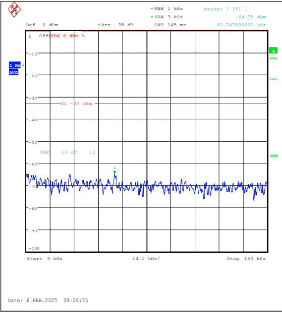
Band26(824-849)-1.4MHz-QPSK-26797-6RB#0-0. 009~0.15-PASS
