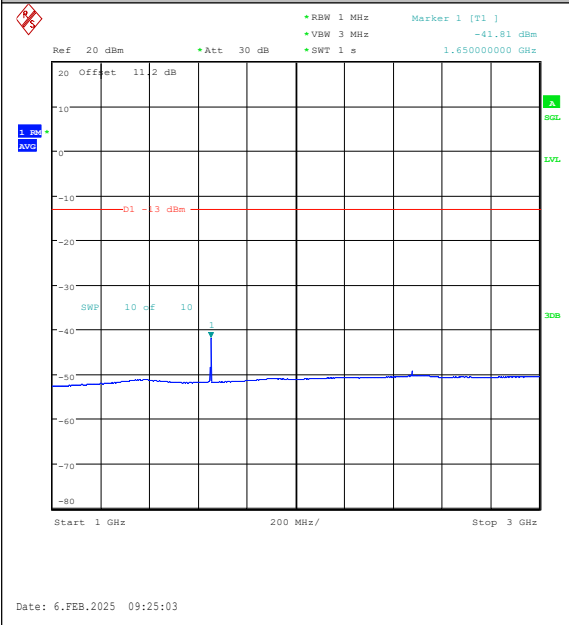
Band26(824-849)-1.4MHz-QPSK-26797-1RB#5-1 000~3000-PASS
