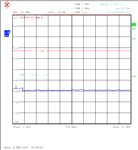
Band26(824-849)-1.4MHz-QPSK-26797-6RB#0-3 000~10000-PASS
