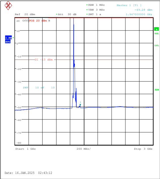
Band2-20MHz-16QAM-18700-1RB#0-1000~3000 -PASS
