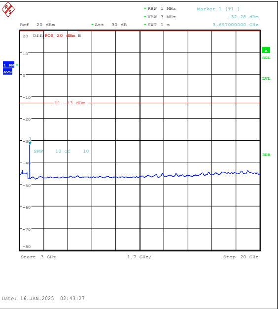
Band2-20MHz-16QAM-18700-1RB#0-3000~20000 -PASS
