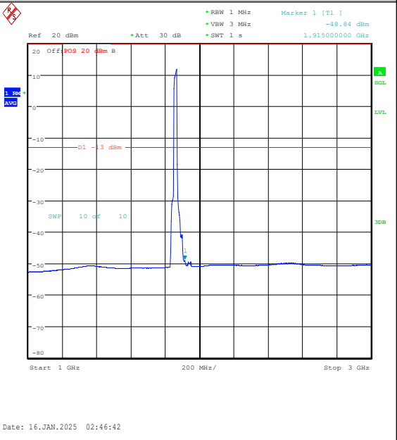
Band2-20MHz-QPSK-18700-100RB#0-1000~3000 -PASS
