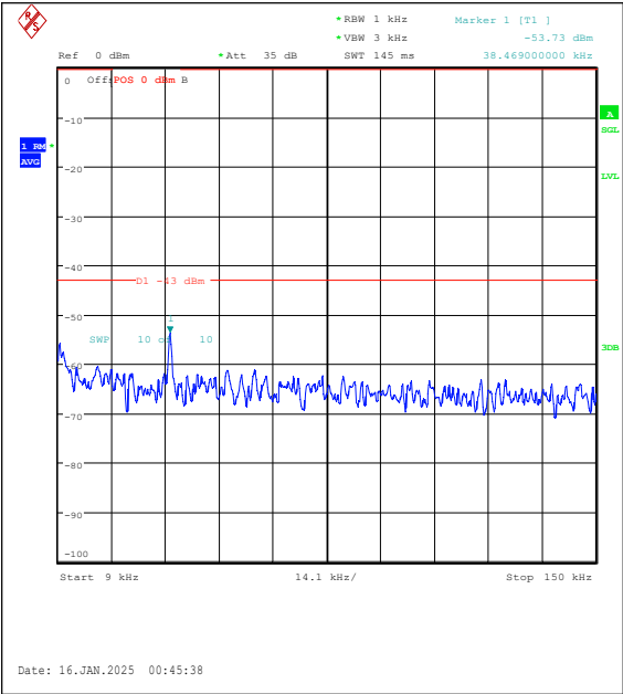
Band2-10MHz-QPSK-18650-50RB#0-0.009~0.15 -PASS
