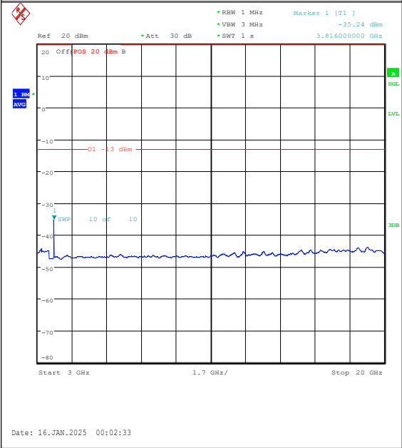
Band2-5MHz-QPSK-19175-25RB#0-3000~20000 -PASS
