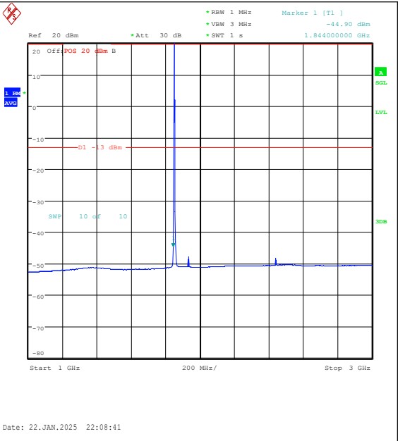
Band25-3MHz-QPSK-26055-1RB#0-1000~3000-P ASS
