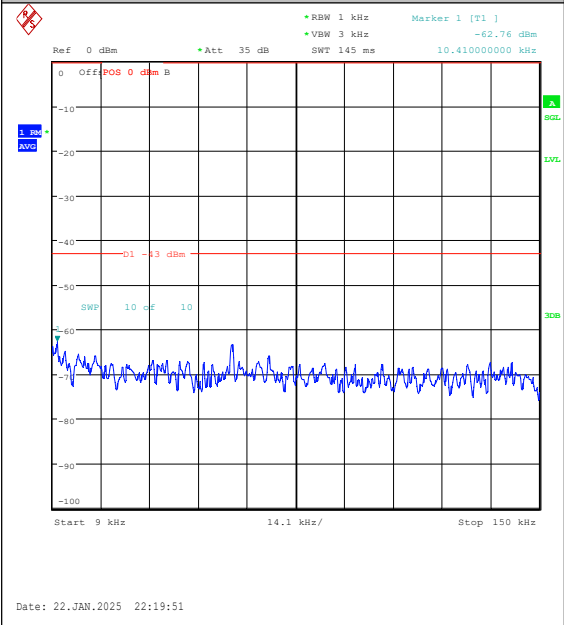
Band25-3MHz-QPSK-26365-15RB#0-0.009~0.15 -PASS
