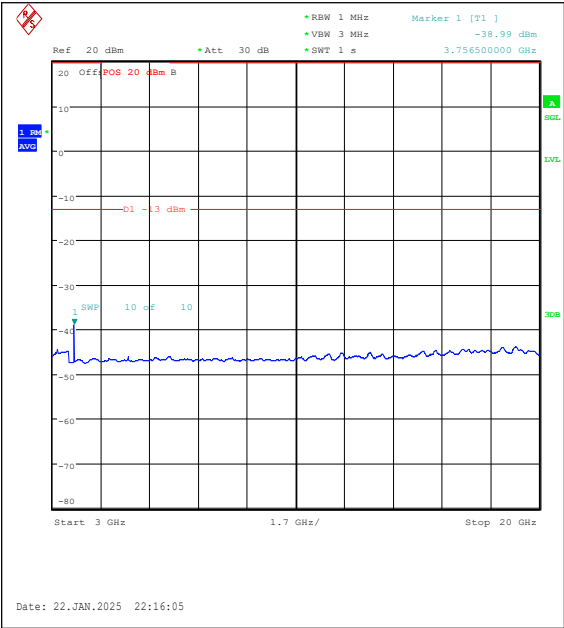
Band25-3MHz-QPSK-26365-1RB#0-3000~20000 -PASS
