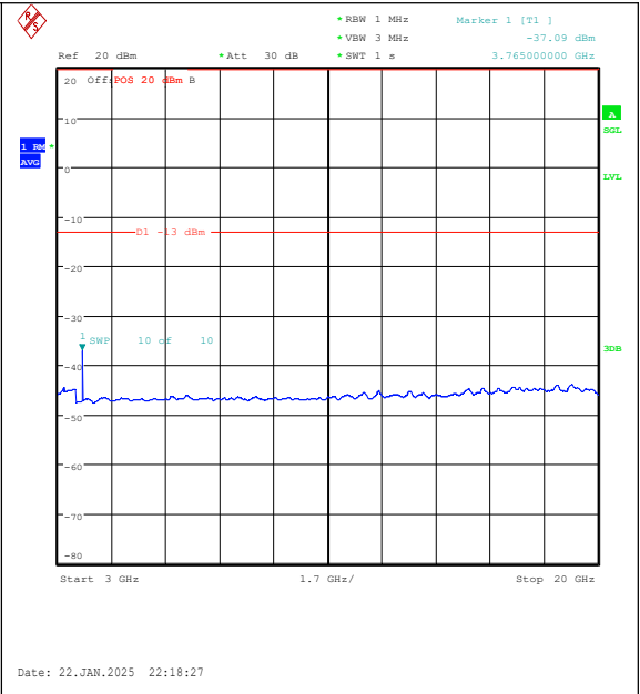
Band25-3MHz-QPSK-26365-1RB#14-3000~20000 -PASS
