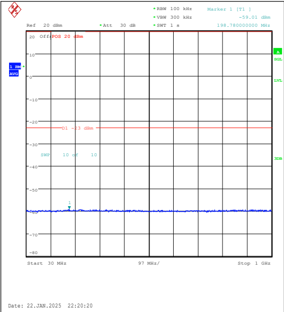
Band25-3MHz-QPSK-26365-15RB#0-30~1000-P ASS
