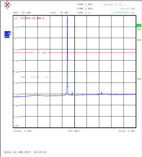
Band25-3MHz-QPSK-26365-1RB#14-1000~3000 -PASS
