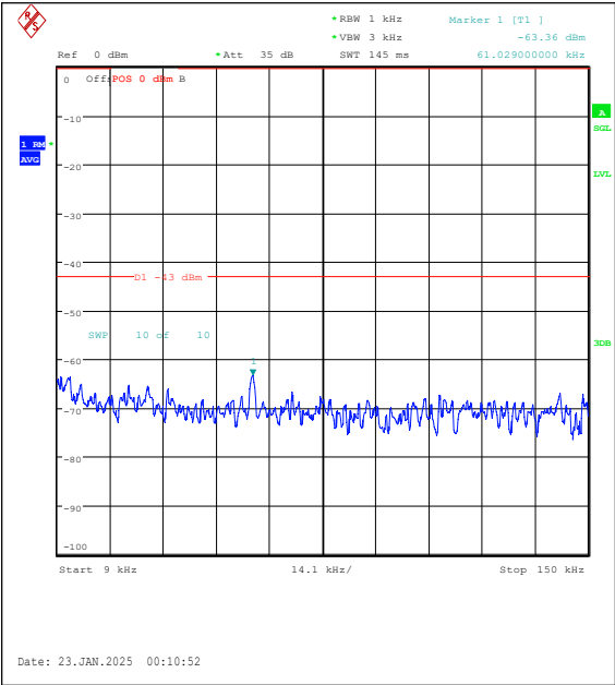
Band25-10MHz-QPSK-26365-1RB#0-0.009~0.15 -PASS
