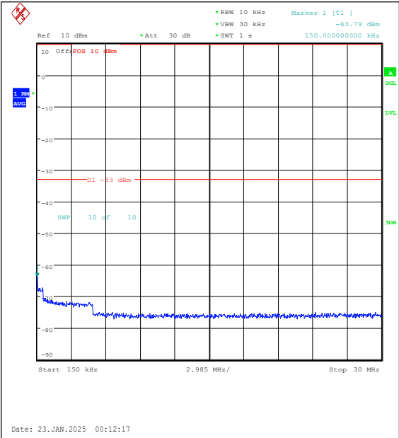
Band25-10MHz-16QAM-26365-1RB#0-0.15~30-P ASS
