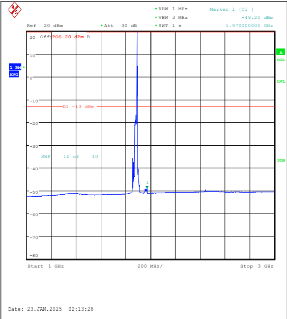
Band25-20MHz-QPSK-26365-1RB#99-1000~300 0-PASS
