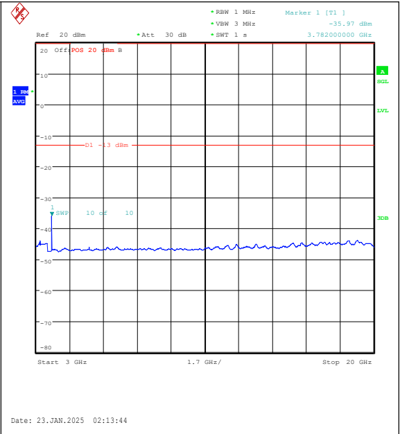
Band25-20MHz-QPSK-26365-1RB#99-3000~2000 0-PASS
