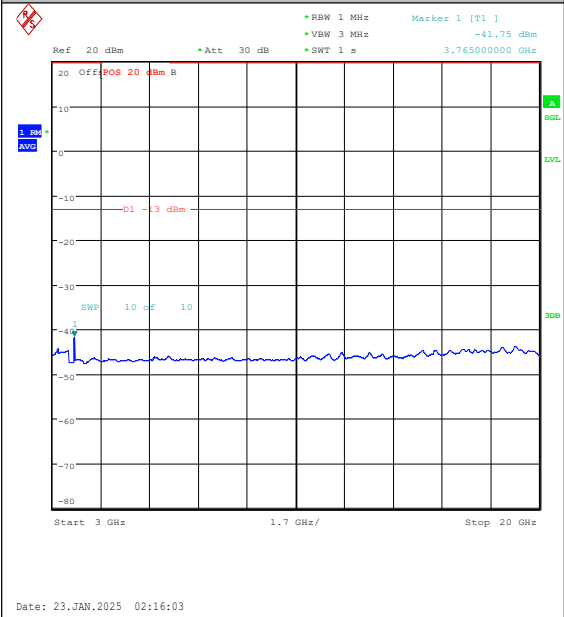
Band25-20MHz-QPSK-26365-100RB#0-3000~20 000-PASS
