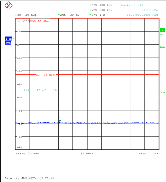
Band25-20MHz-16QAM-26590-1RB#99-30~1000 -PASS
