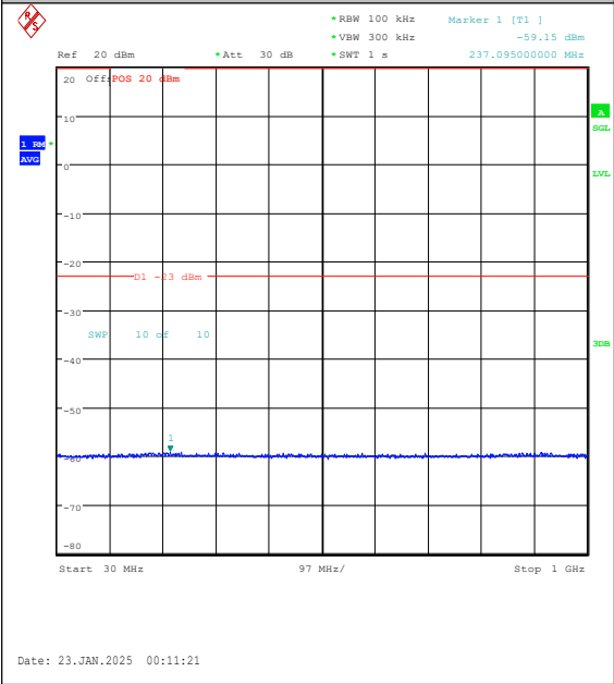
Band25-10MHz-QPSK-26365-1RB#0-30~1000-P ASS
