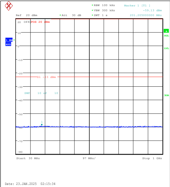
Band25-20MHz-QPSK-26365-100RB#0-30~1000 -PASS
