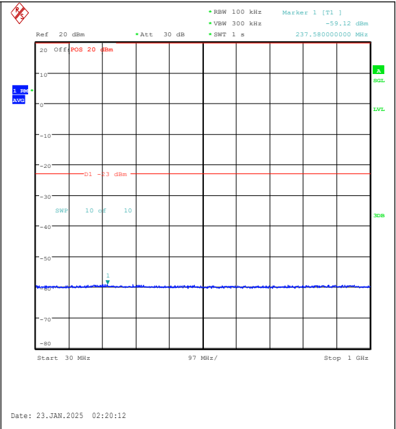
Band25-20MHz-QPSK-26590-1RB#99-30~1000-P ASS
