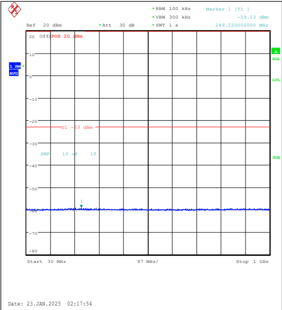
Band25-20MHz-QPSK-26590-1RB#0-30~1000-P ASS
