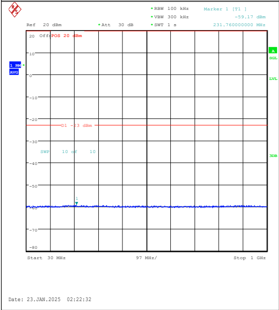
Band25-20MHz-QPSK-26590-100RB#0-30~1000 -PASS
