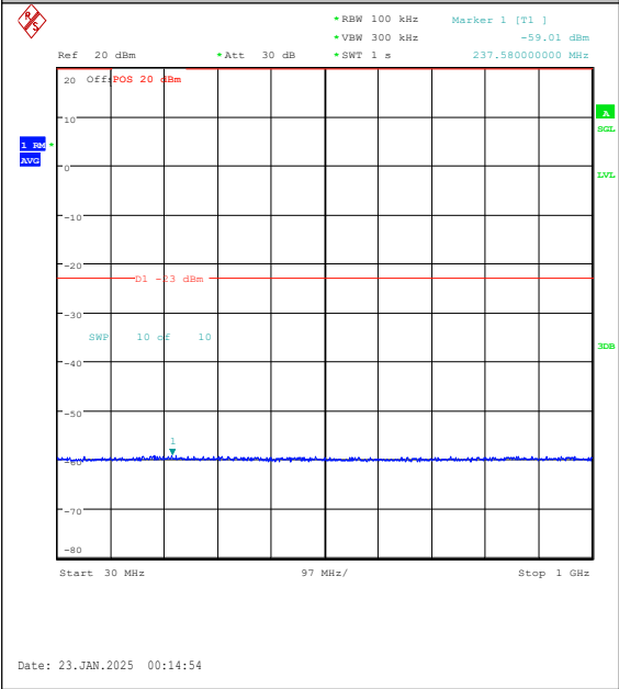
Band25-10MHz-16QAM-26365-1RB#49-30~1000 -PASS
