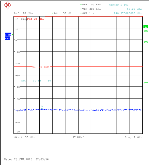
Band25-20MHz-QPSK-26140-1RB#0-30~1000-P ASS
