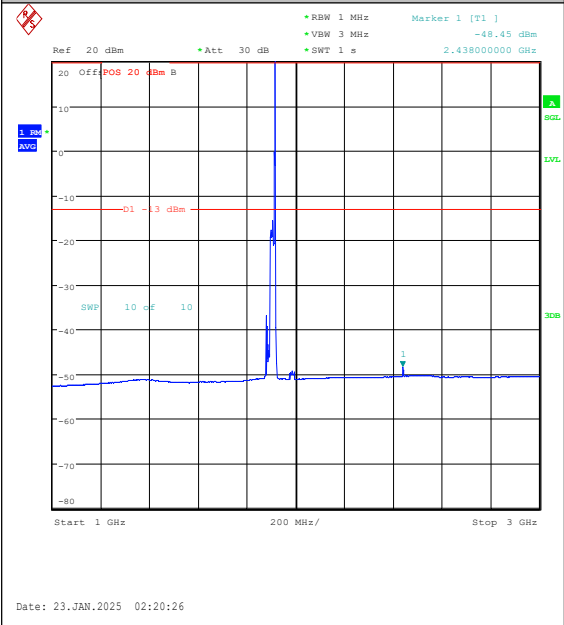
Band25-20MHz-QPSK-26590-1RB#99-1000~300 0-PASS
