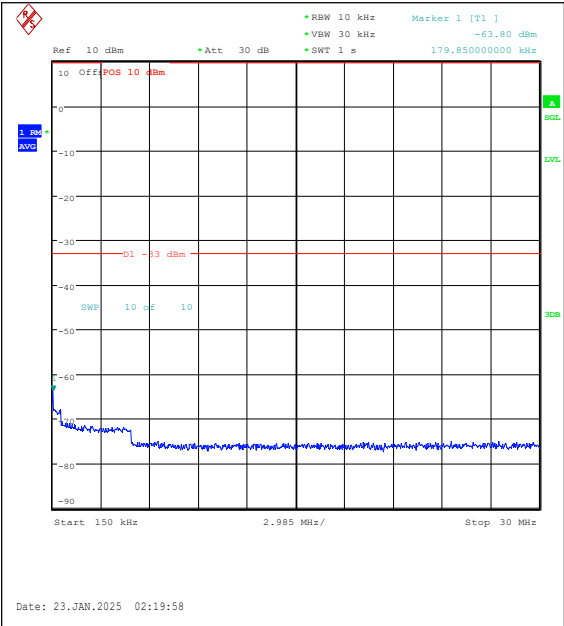
Band25-20MHz-QPSK-26590-1RB#99-0.15~30-P ASS
