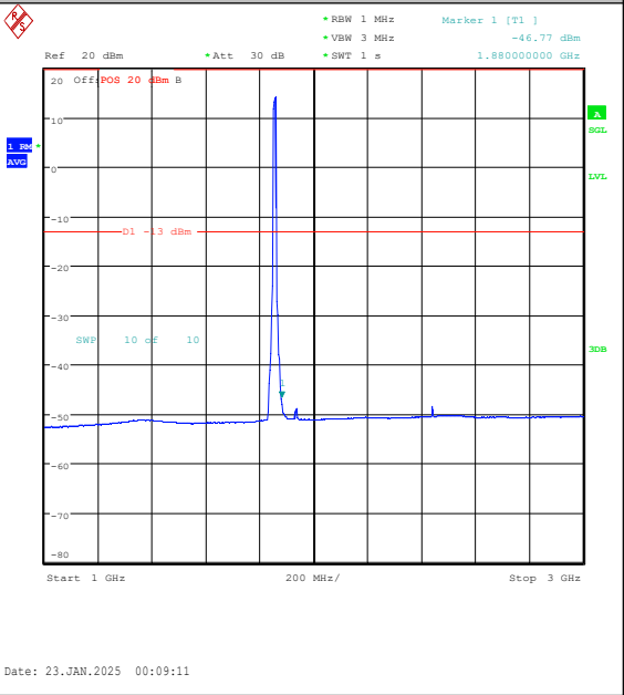
Band25-10MHz-QPSK-26090-50RB#0-1000~3000 -PASS
