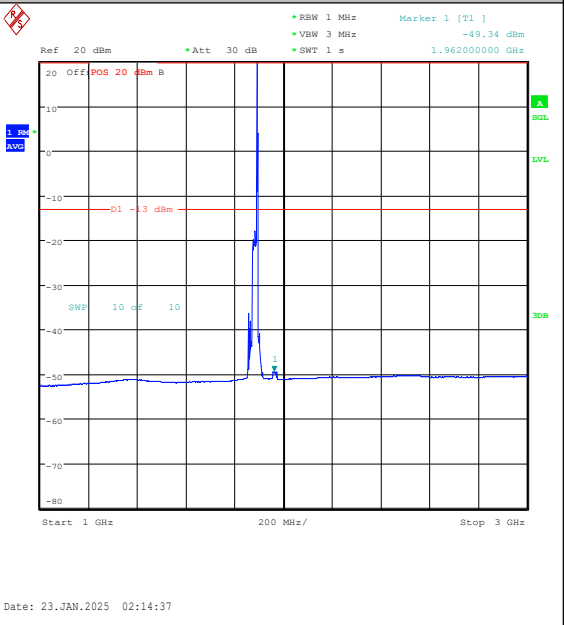
Band25-20MHz-16QAM-26365-1RB#99-1000~3000-PASS
