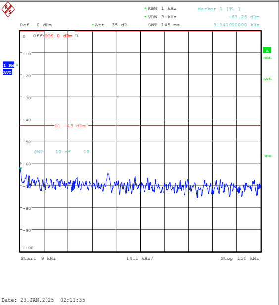
Band25-20MHz-16QAM-26365-1RB#0-0.009~0.15 -PASS
