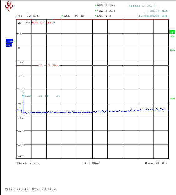
Band25-5MHz-QPSK-26365-1RB#0-3000~20000 -PASS
