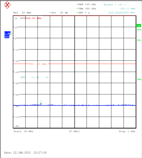
Band25-3MHz-QPSK-26675-15RB#0-30~1000-P ASS
