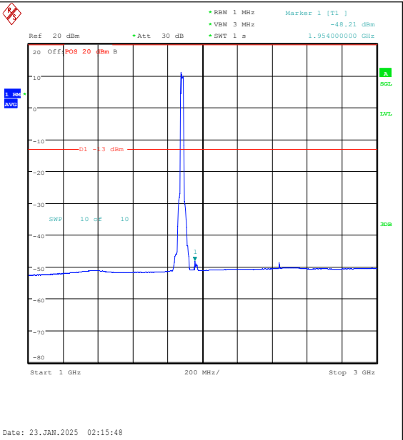
Band25-20MHz-QPSK-26365-100RB#0-1000~300 0-PASS
