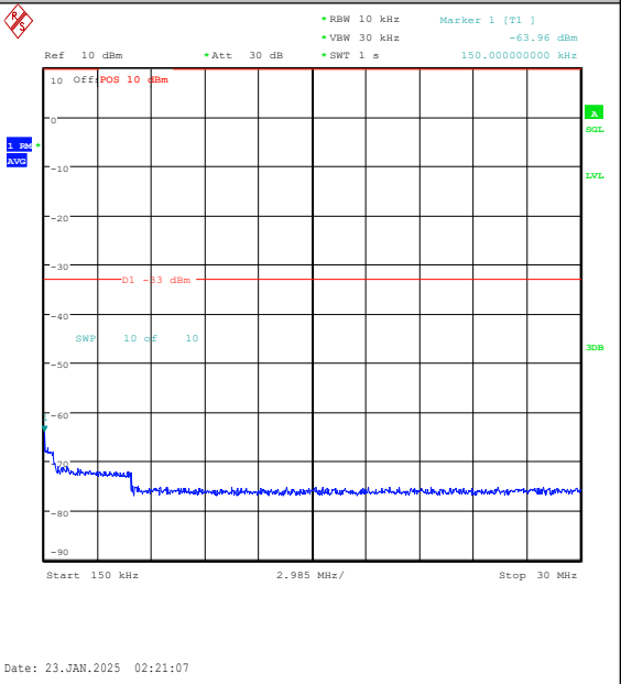
Band25-20MHz-16QAM-26590-1RB#99-0.15~30-P ASS
