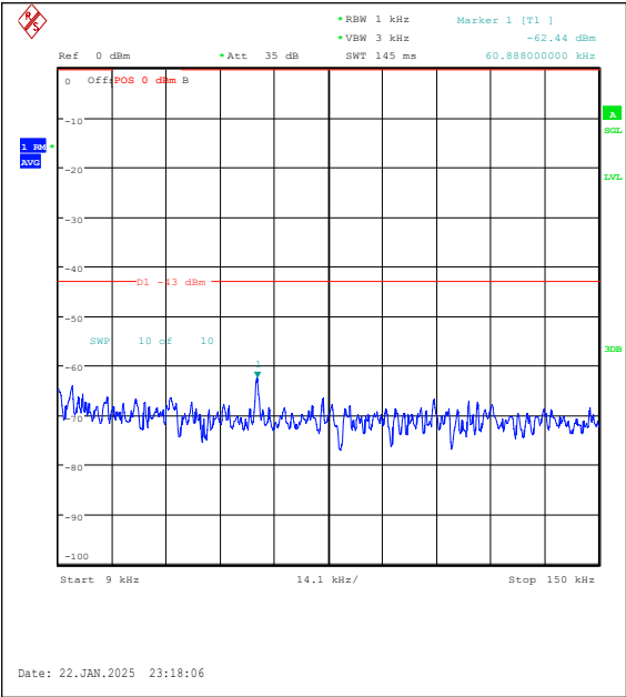
Band25-5MHz-QPSK-26365-25RB#0-0.009~0.15 -PASS
