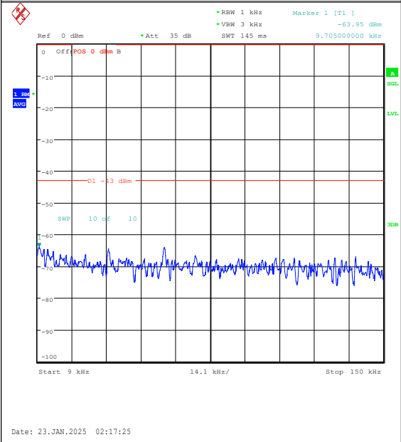
Band25-20MHz-QPSK-26590-1RB#0-0.009~0.15 -PASS
