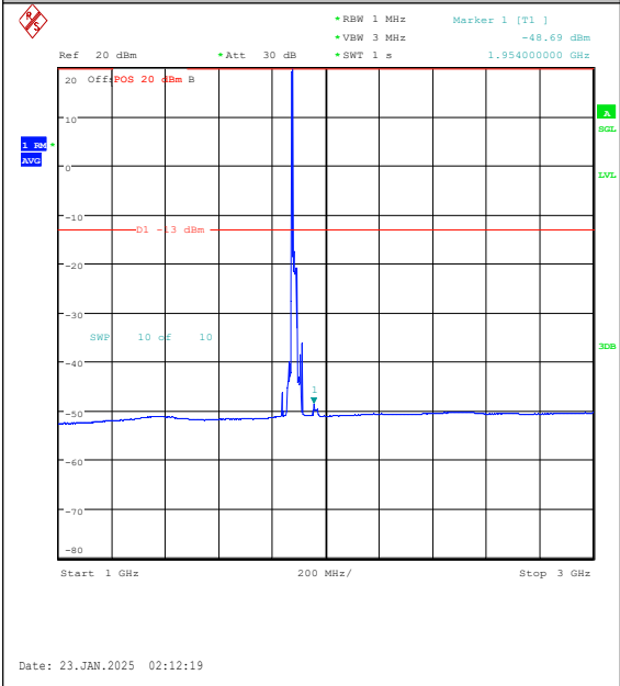
Band25-20MHz-16QAM-26365-1RB#0-1000~300 0-PASS
