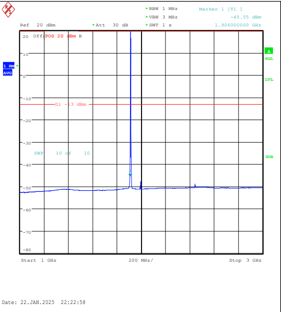
Band25-3MHz-QPSK-26675-1RB#0-1000~3000-P ASS
