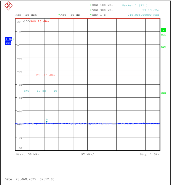
Band25-20MHz-16QAM-26365-1RB#0-30~1000-P ASS
