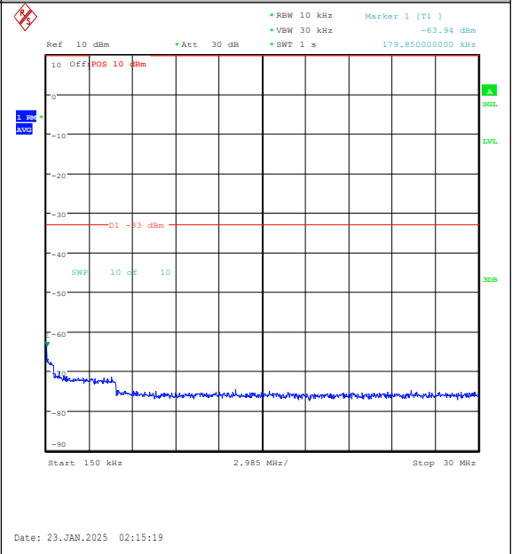
Band25-20MHz-QPSK-26365-100RB#0-0.15~30-P ASS
