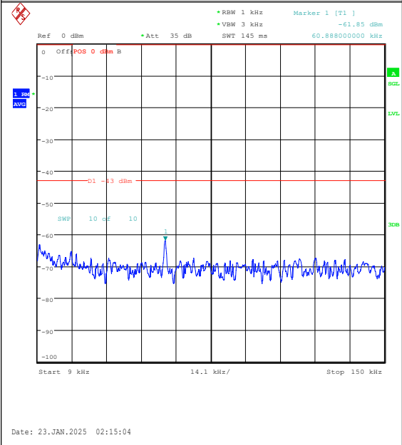
Band25-20MHz-QPSK-26365-100RB#0-0.009~0. 15-PASS
