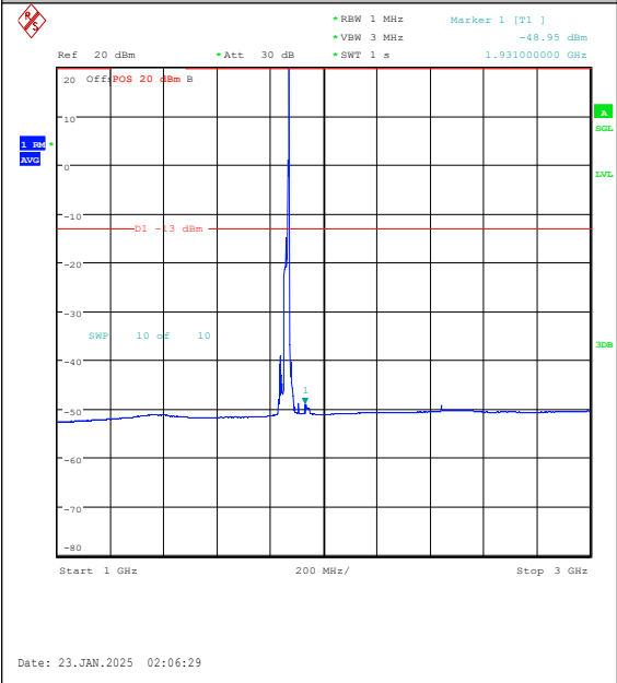
Band25-20MHz-QPSK-26140-1RB#99-1000~300 0-PASS
