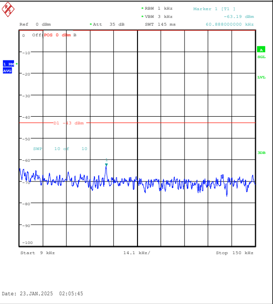
Band25-20MHz-QPSK-26140-1RB#99-0.009~0.15 -PASS
