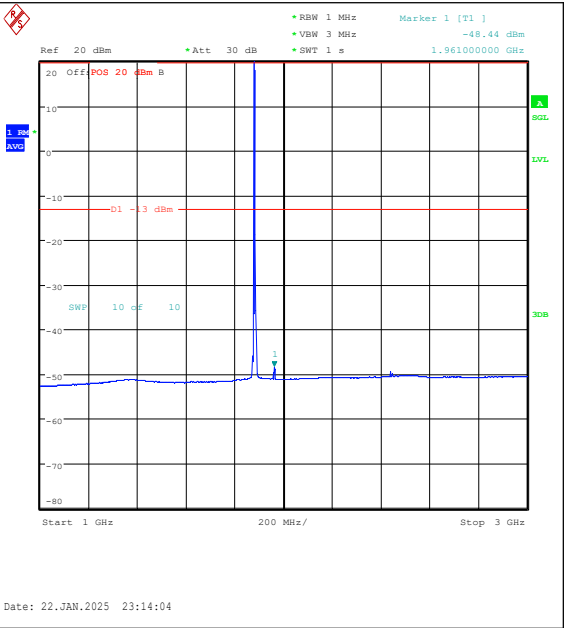
Band25-5MHz-QPSK-26365-1RB#0-1000~3000-P ASS
