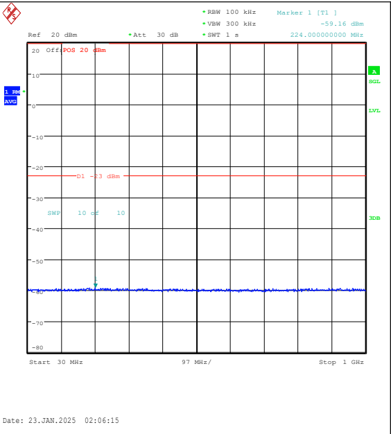
Band25-20MHz-QPSK-26140-1RB#99-30~1000-P ASS
