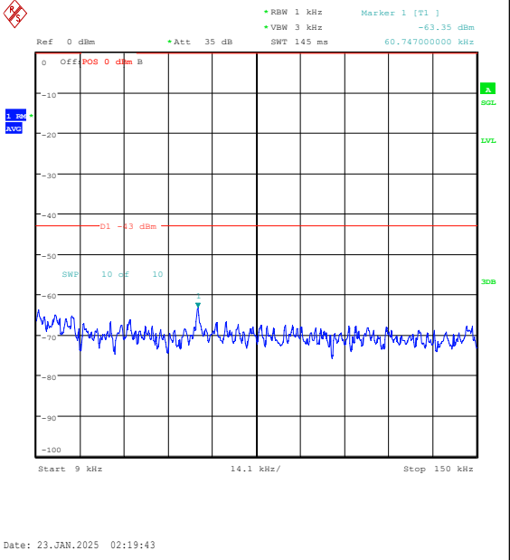
Band25-20MHz-QPSK-26590-1RB#99-0.009~0.15 -PASS
