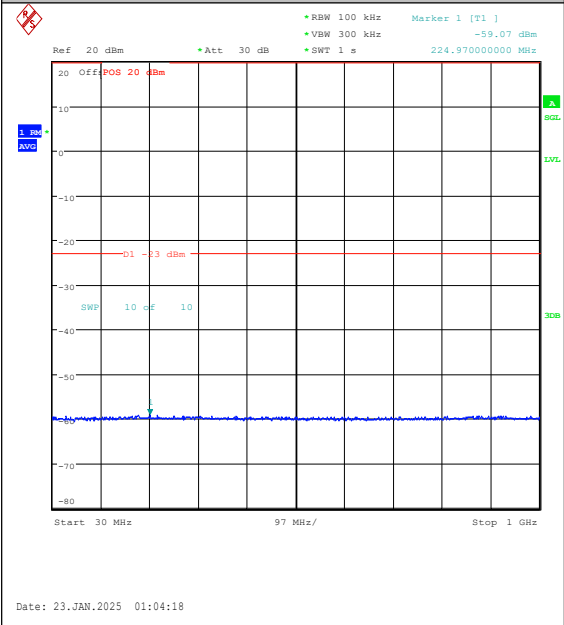
Band25-15MHz-QPSK-26115-1RB#0-30~1000-P ASS
