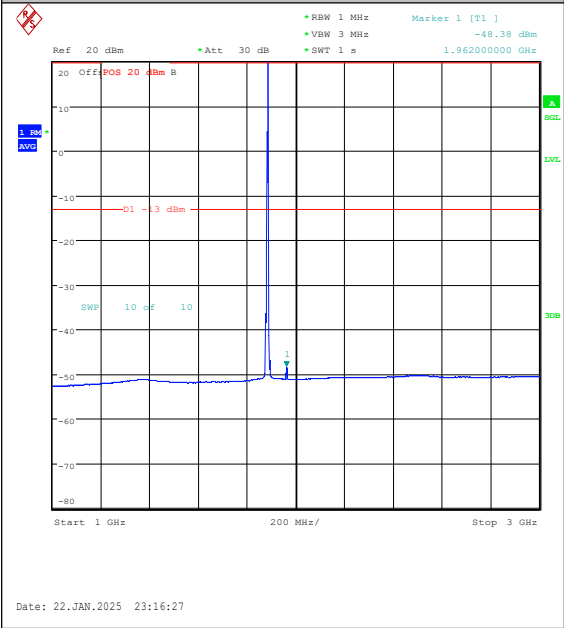
Band25-5MHz-QPSK-26365-1RB#24-1000~3000 -PASS
