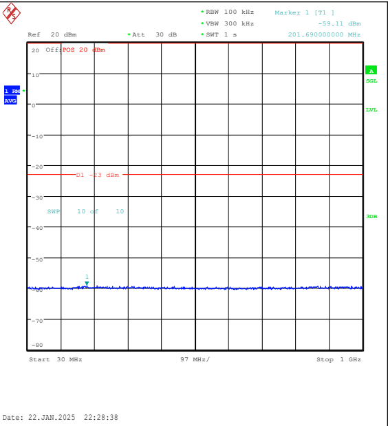
Band25-3MHz-16QAM-26675-15RB#0-30~1000-P ASS
