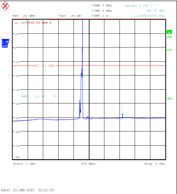
Band25-20MHz-16QAM-26590-1RB#99-1000~300 0-PASS
