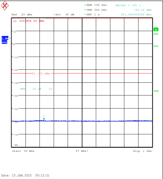
Band25-10MHz-16QAM-26365-1RB#0-30~1000-P ASS
