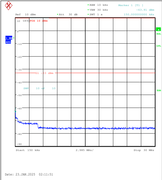
Band25-20MHz-16QAM-26365-1RB#0-0.15~30-P ASS
