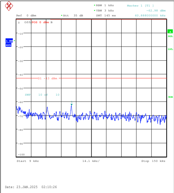
Band25-20MHz-QPSK-26365-1RB#0-0.009~0.15 -PASS
