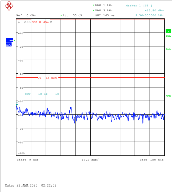
Band25-20MHz-QPSK-26590-100RB#0-0.009~0. 15-PASS
