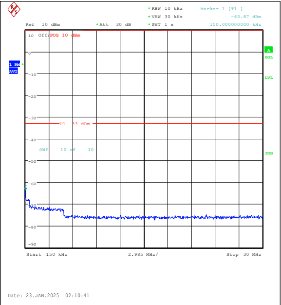
Band25-20MHz-QPSK-26365-1RB#0-0.15~30-PA SS
