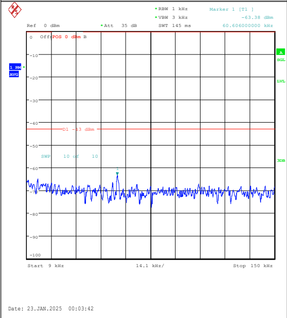
Band25-10MHz-QPSK-26090-1RB#0-0.009~0.15 -PASS
