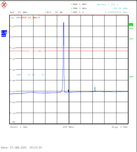
Band25-10MHz-QPSK-26640-50RB#0-1000~3000 -PASS
