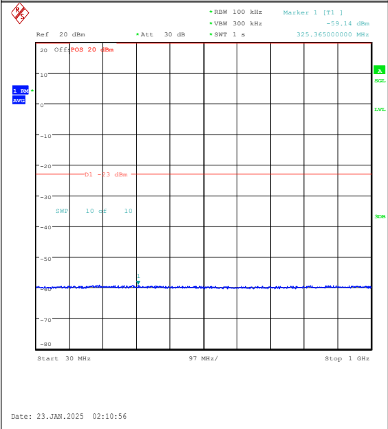
Band25-20MHz-QPSK-26365-1RB#0-30~1000-P ASS
