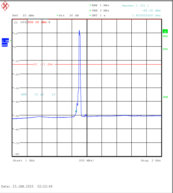
Band25-20MHz-QPSK-26590-100RB#0-1000~300 0-PASS
