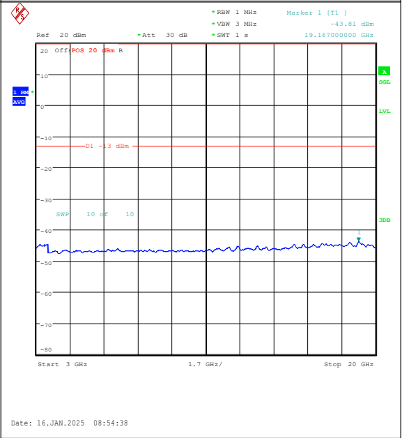
Band4-10MHz-QPSK-20000-1RB#49-3000~20000 -PASS
