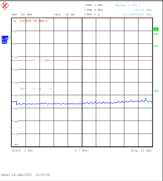
Band4-20MHz-QPSK-20050-1RB#99-3000~20000 -PASS
