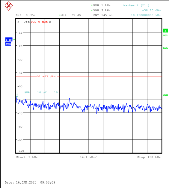
Band4-10MHz-QPSK-20175-50RB#0-0.009~0.15 -PASS
