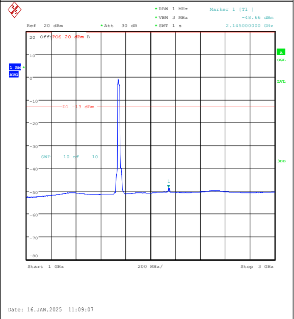
Band4-20MHz-QPSK-20300-100RB#0-1000~3000 -PASS
