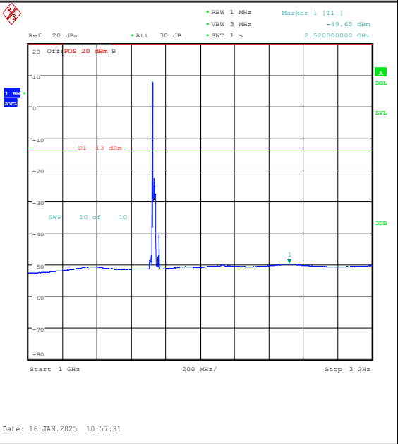
Band4-20MHz-QPSK-20175-1RB#0-1000~3000-P ASS
