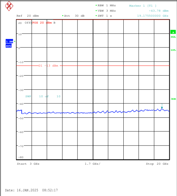
Band4-10MHz-QPSK-20000-1RB#0-3000~20000 -PASS
