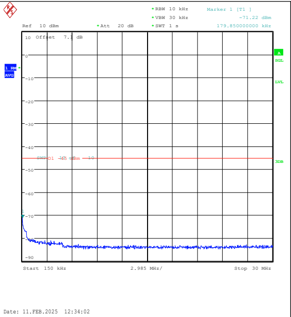
Band41(2535-2655)-20MHz-QPSK-40590-1RB#0- 0.15~30-PASS
