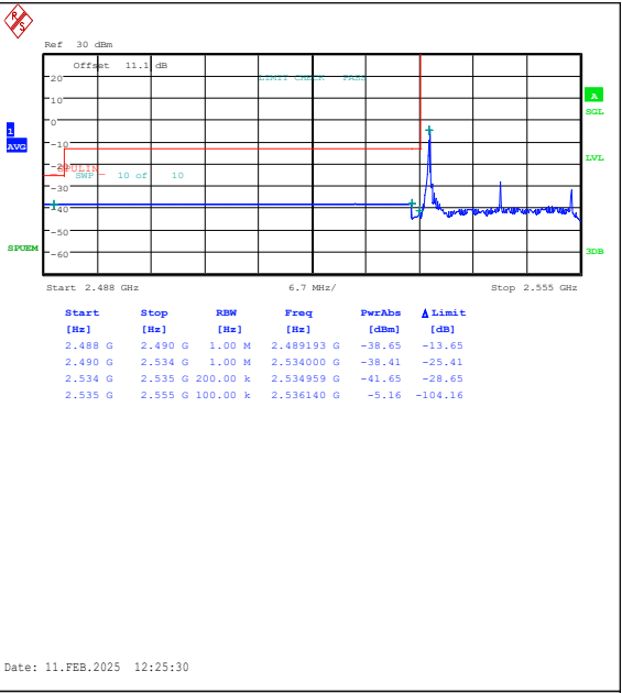
Band41(2535-2655)-20MHz-16QAM-40140-1RB#0 -PASS
