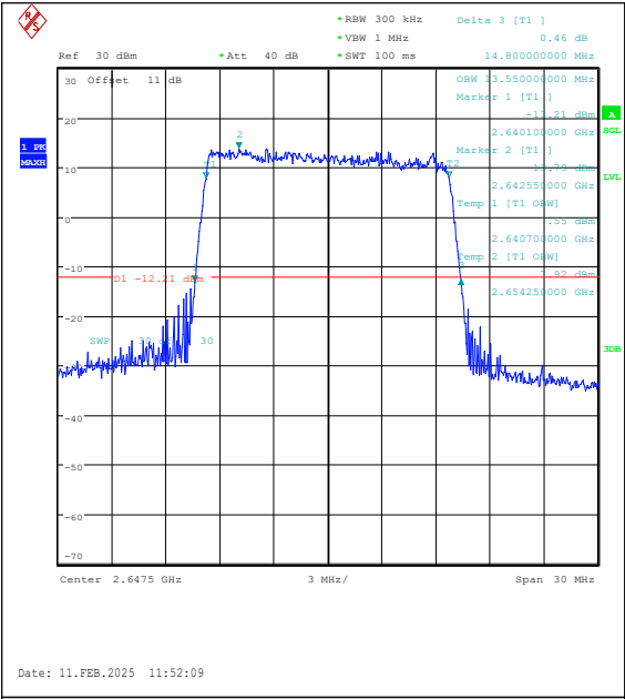
Band41(2535-2655)-15MHz-QPSK-41165-75RB# 0-PASS
