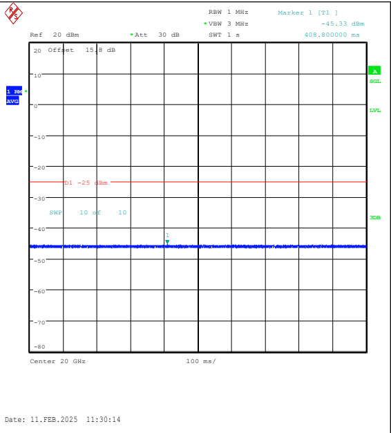
Band41(2535-2655)-10MHz-16QAM-40590-1RB# -20000~27000-PASS
