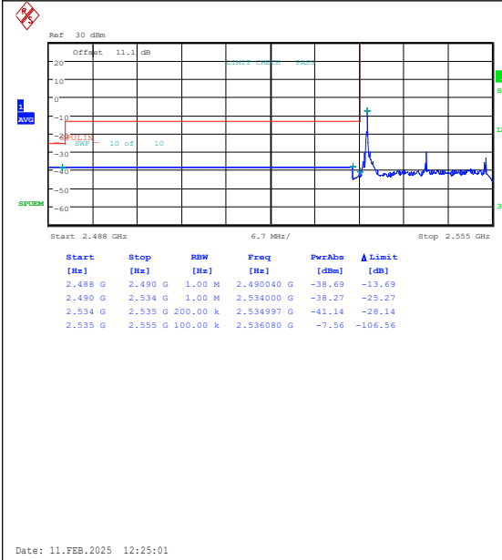
Band41(2535-2655)-20MHz-QPSK-40140-1RB#0 -PASS
