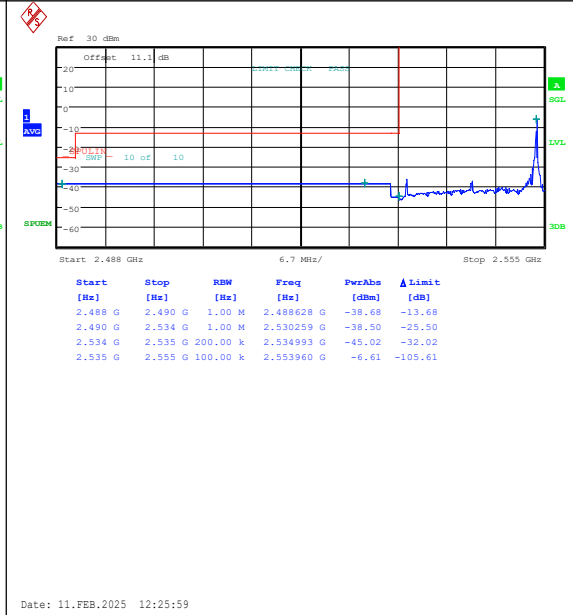
Band41(2535-2655)-20MHz-QPSK-40140-1RB#99 -PASS
