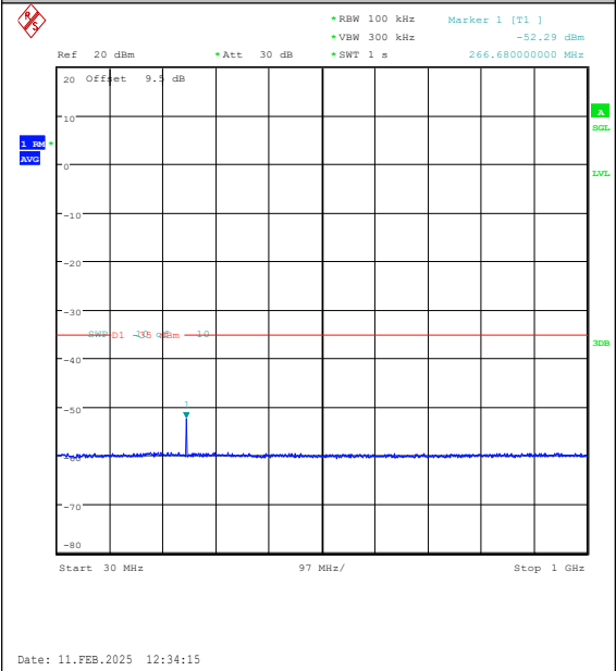
Band41(2535-2655)-20MHz-QPSK-40590-1RB#0 -30~1000-PASS
