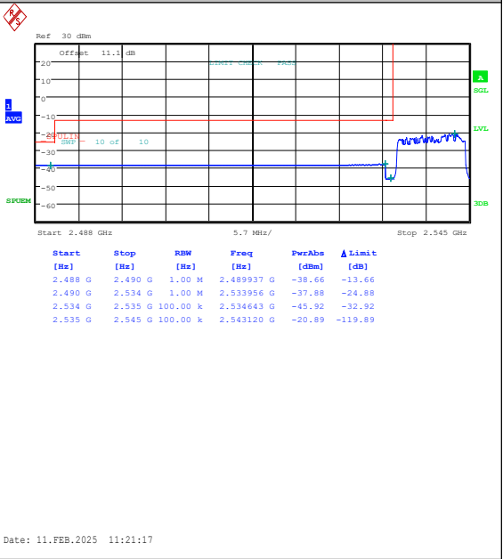
Band41(2535-2655)-10MHz-16QAM-40090-50RB# 0-PASS
