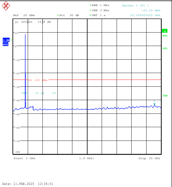
Band41(2535-2655)-20MHz-QPSK-40590-1RB#0- 1000~20000-PASS
