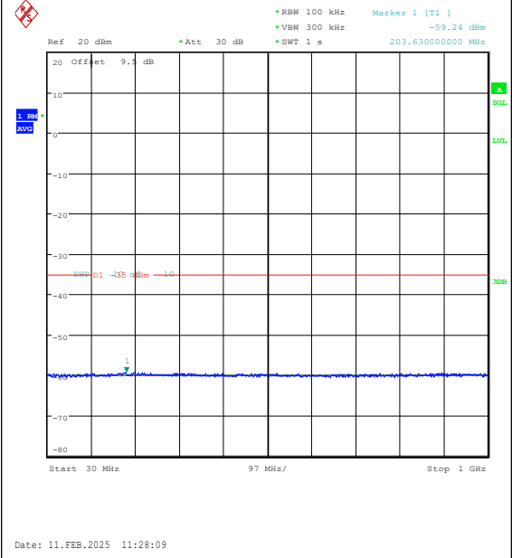
Band41(2535-2655)-10MHz-QPSK-40590-1RB#0 -30~1000-PASS
