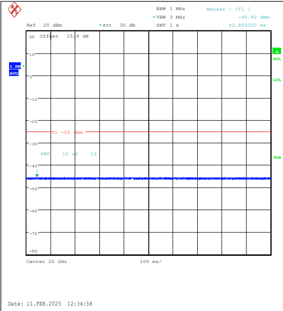
Band41(2535-2655)-20MHz-QPSK-40590-1RB#0 -20000~27000-PASS
