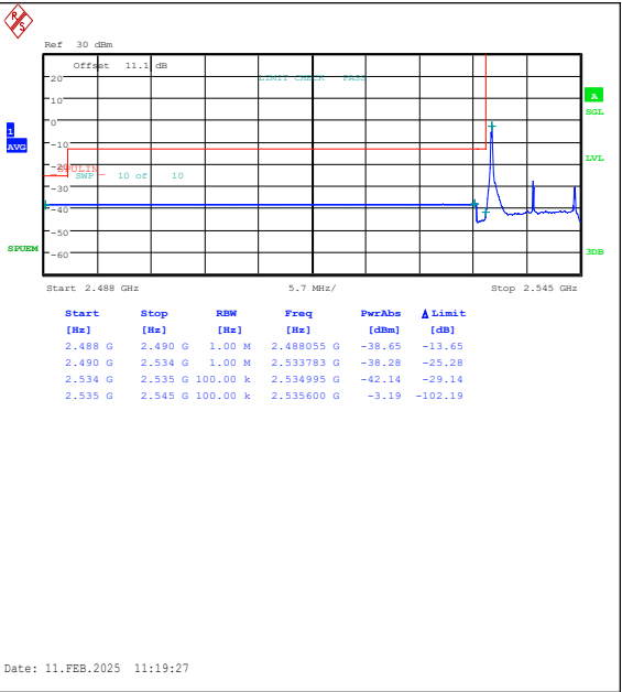
Band41(2535-2655)-10MHz-16QAM-40090-1RB#0 -PASS
