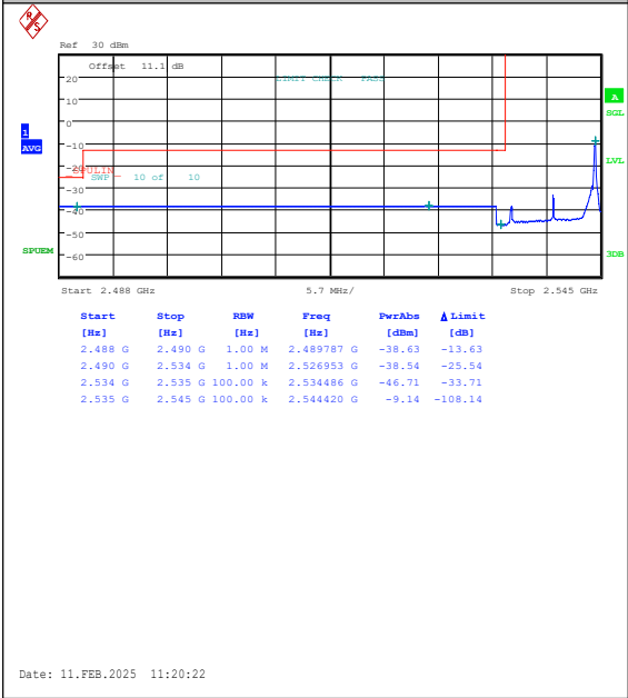
Band41(2535-2655)-10MHz-16QAM-40090-1RB# 49-PASS
