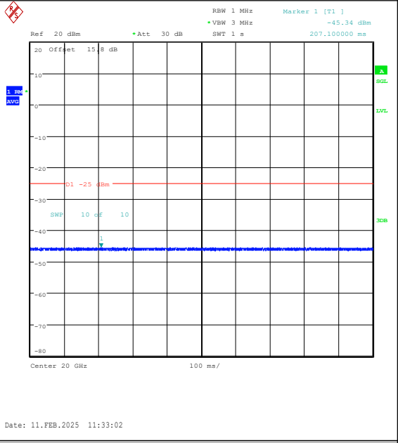
Band41(2535-2655)-10MHz-16QAM-41190-1RB#0 -20000~27000-PASS
