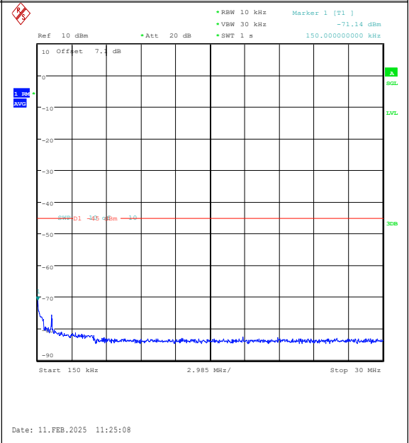
Band41(2535-2655)-10MHz-QPSK-40090-1RB#0- 0.15~30-PASS
