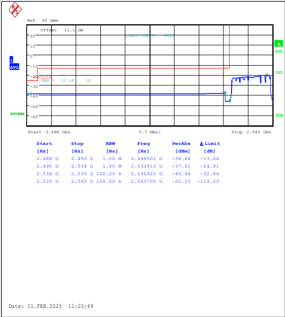
Band41(2535-2655)-10MHz-QPSK-40090-50RB# 0-PASS
