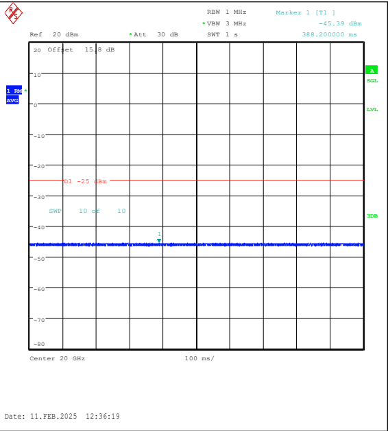
Band41(2535-2655)-20MHz-16QAM-40590-1RB# -20000~27000-PASS
