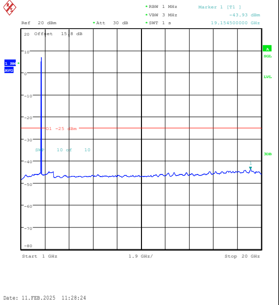
Band41(2535-2655)-10MHz-QPSK-40590-1RB#0- 1000~20000-PASS
