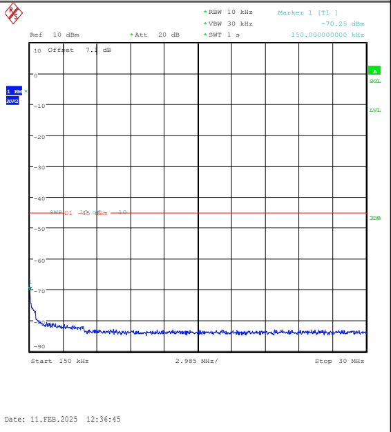
Band41(2535-2655)-20MHz-QPSK-41140-1RB#0- 0.15~30-PASS
