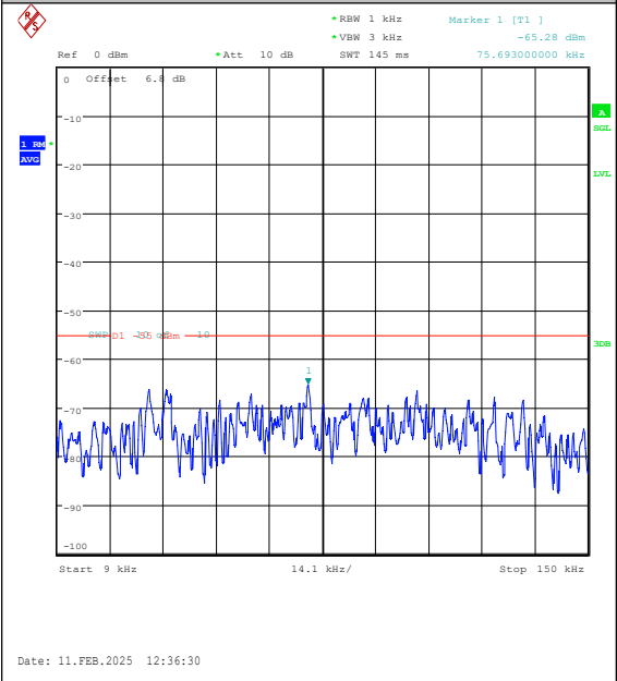
Band41(2535-2655)-20MHz-QPSK-41140-1RB#0- 0.009~0.15-PASS
