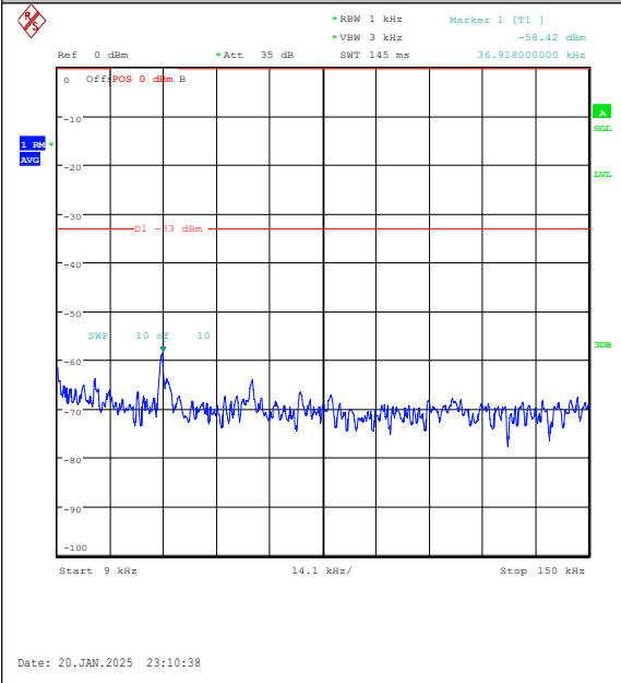
Band5-3MHz-QPSK-20635-15RB#0-0.009~0.15-P ASS
