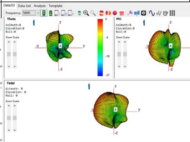
ANT0: 5800Mhz
