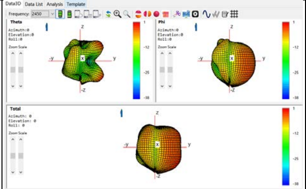
ANT0: 2450Mhz
