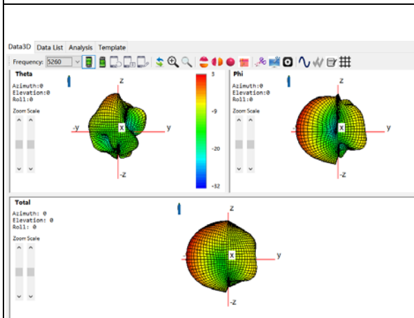
ANT0: 5260Mhz
