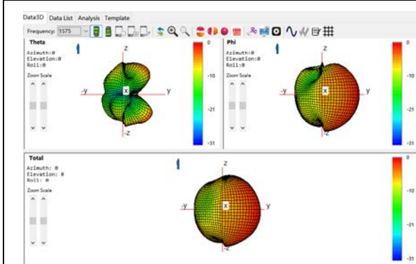
ANT0: 1575Mhz
