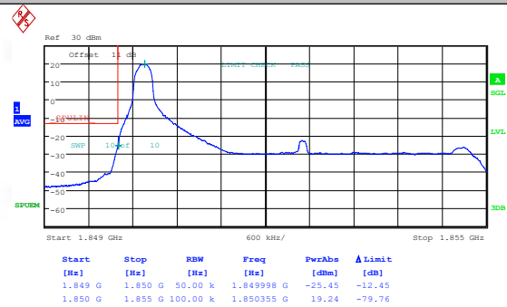
Band2-5MHz-QPSK-18625-1RB#24-PASS
