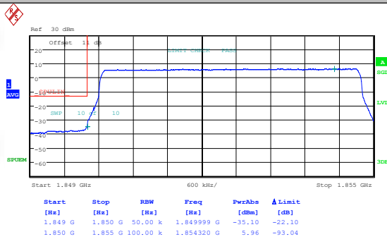
Band2-5MHz-QPSK-18625-1RB#0-PASS
