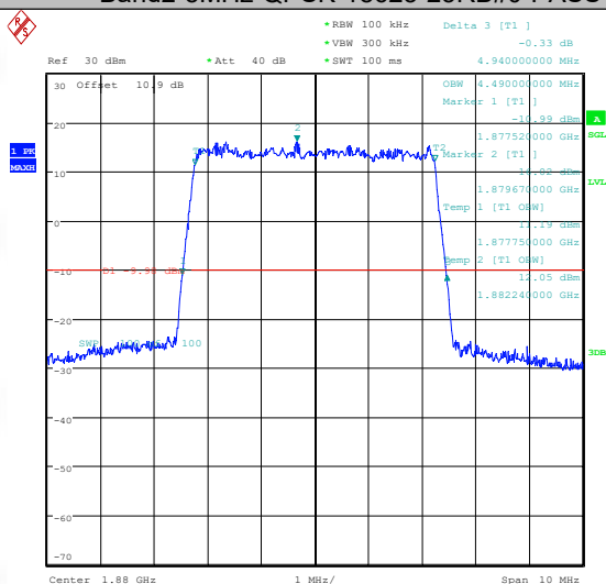
Band2-5MHz-QPSK-18625-25RB#0-PASS
