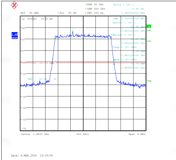
Band25-3MHz-QPSK-26365-15RB#0-PASS
