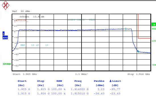
Band25-10MHz-QPSK-26640-1RB#0-PASS
