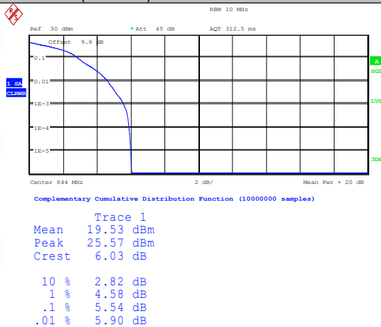
Band26(824-849)-10MHz-QPSK-26990-1RB#0-PASS
