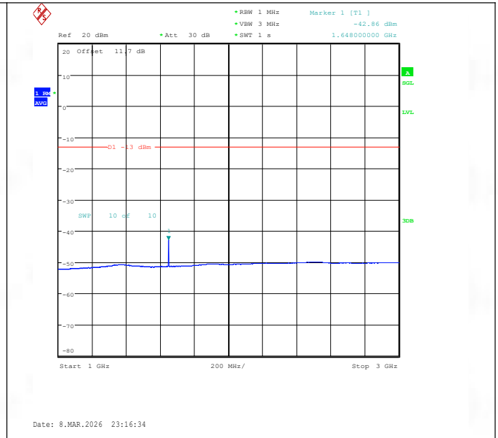
Band26(824-849)-3MHz-QPSK-26805-1RB#0-1000~3000-PASS
