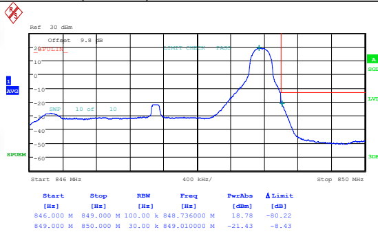
Band26(824-849)-3MHz-QPSK-27025-15RB#0-PASS
