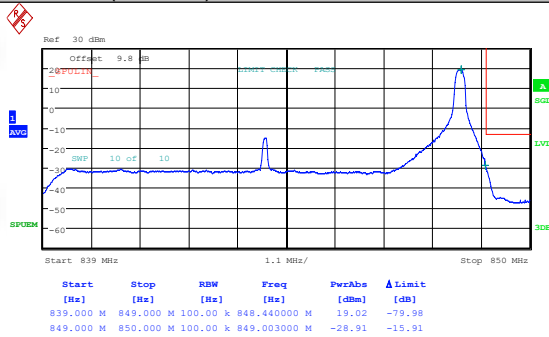
Band26(824-849)-10MHz-QPSK-26990-50RB#0-PASS
