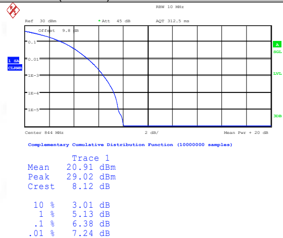
Band26(824-849)-10MHz-QPSK-26990-50RB#0-PASS
