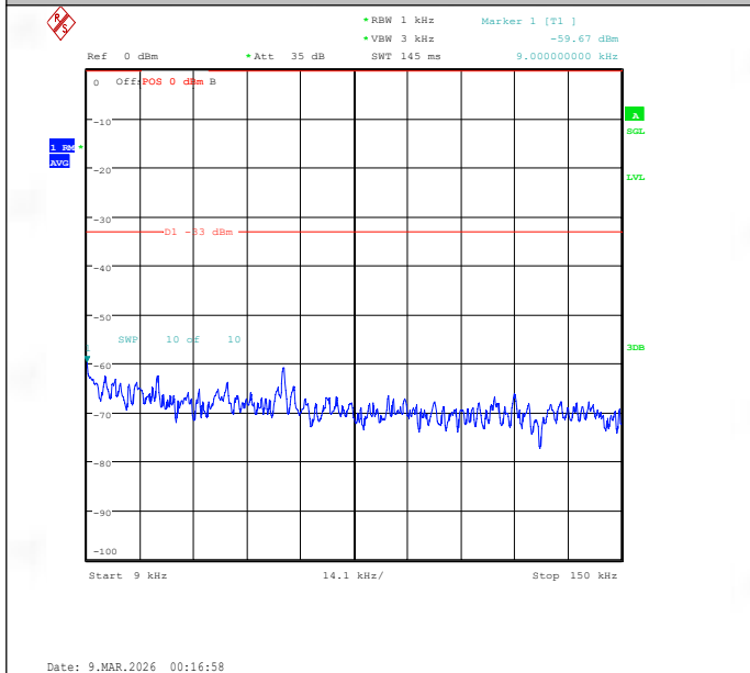
Band26(824-849)-10MHz-QPSK-26990-1RB#0-0.009~0.15-PASS
