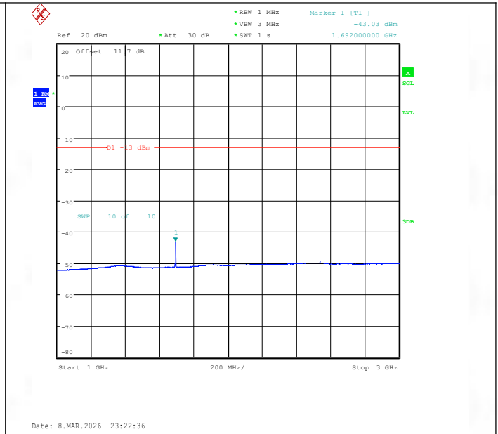
Band26(824-849)-3MHz-QPSK-27025-1RB#0-1000~3000-PASS
