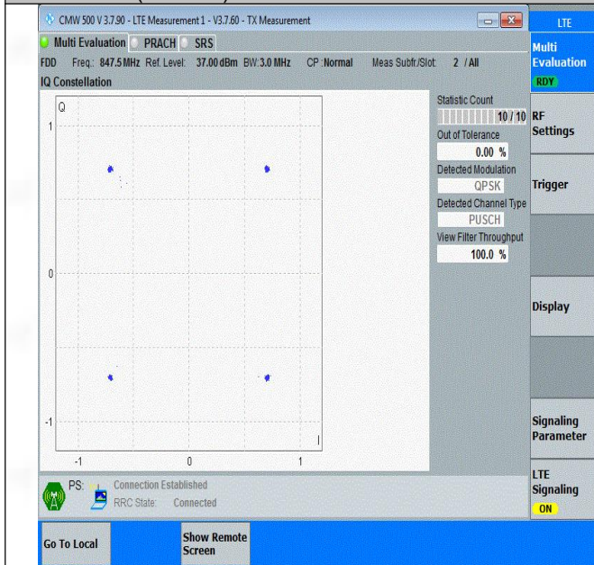
Band26(824-849)-3MHz-QPSK-27025-15RB#0-PASS
