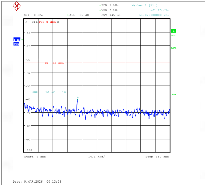
Band26(824-849)-10MHz-QPSK-26915-1RB#0-0.009~0.15-PASS
