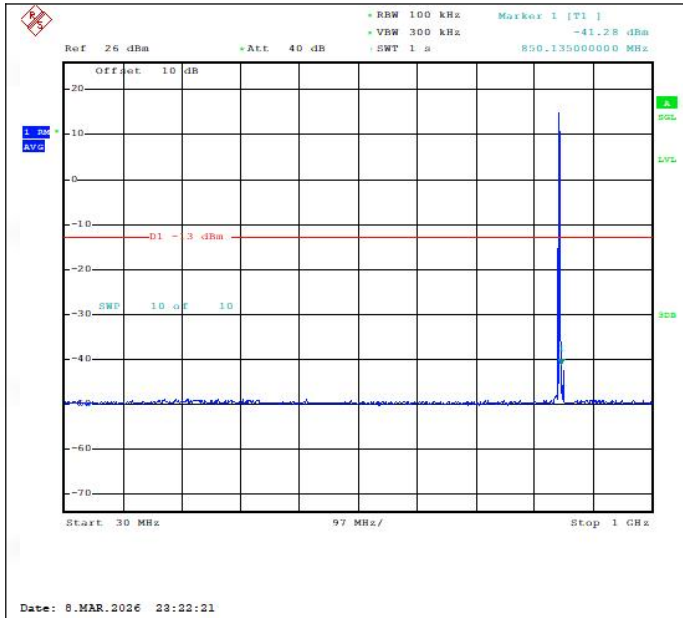
Band26(824-849)-3MHz-QPSK-27025-1RB#0-30~1000-PASS
