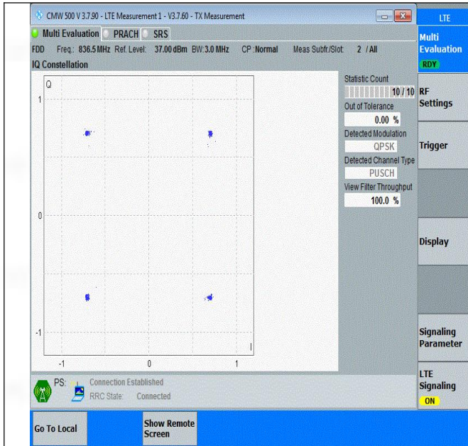
Band26(824-849)-3MHz-QPSK-26915-15RB#0-PASS
