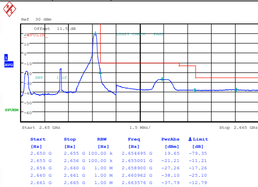
Band41(2535-2655)-5MHz-QPSK-41215-25RB#0-PASS
