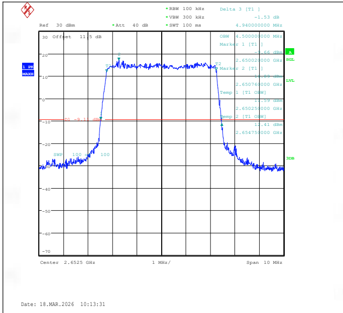
Band41(2535-2655)-5MHz-QPSK-41215-25RB#0-PASS
