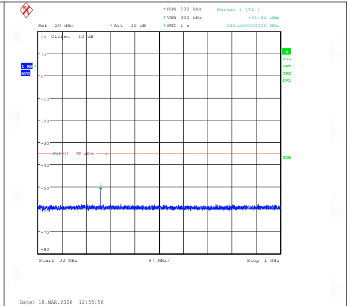
Band41(2535-2655)-10MHz-QPSK-40590-1RB#49-30~1000-PASS
