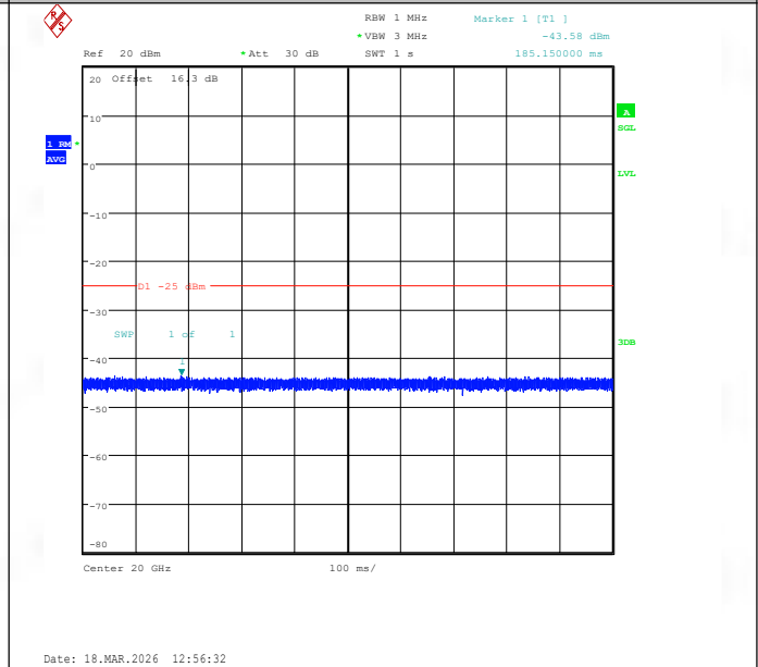
Band41(2535-2655)-10MHz-QPSK-40590-1RB#49-20000~27000-PASS
