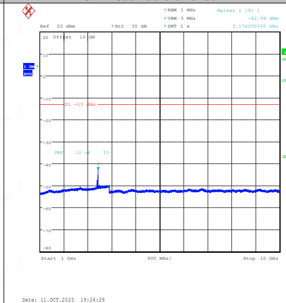
EGPRS850-190-8-1000~10000MHz-PASS
