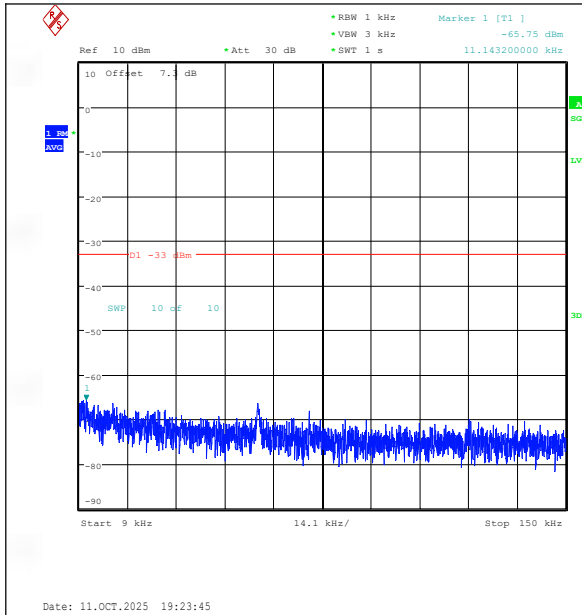
EGPRS850-190-8-0.009~0.15MHz-PASS
