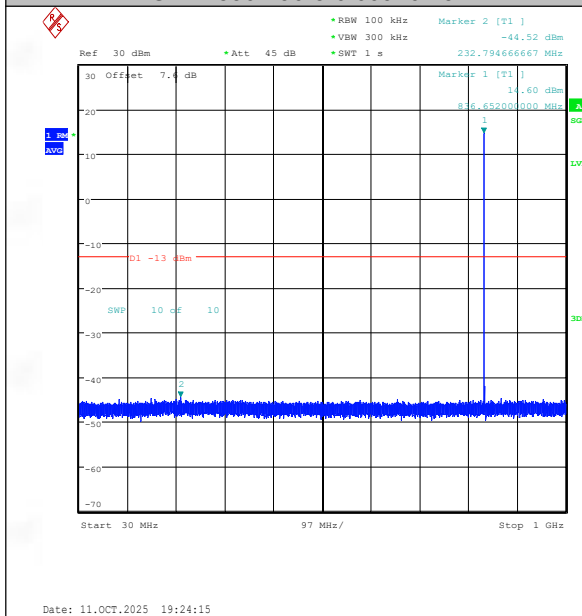
EGPRS850-190-8-30~1000MHz-PASS
