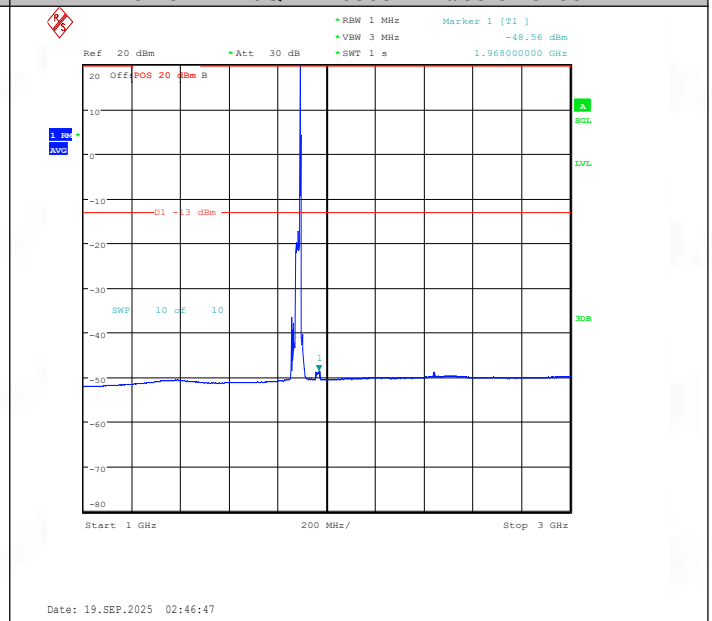
Band25-20MHz-16QAM-26365-1RB#99-1000~3000-PASS
