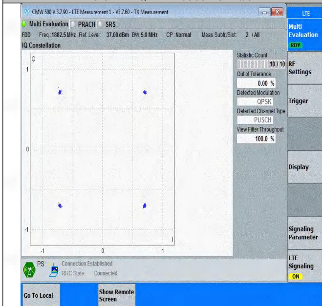
Band25-5MHz-QPSK-26365-25RB#0-PASS
