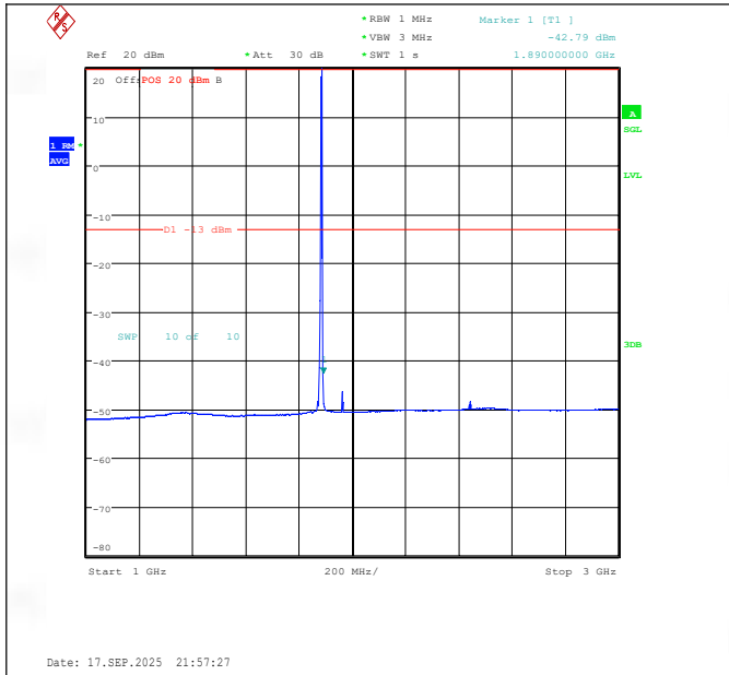
Band25-3MHz-QPSK-26365-1RB#14-1000~3000-PASS
