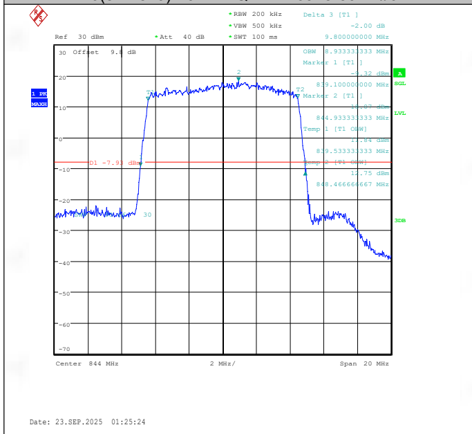
Band26(824-849)-10MHz-QPSK-26990-50RB#0-PASS
