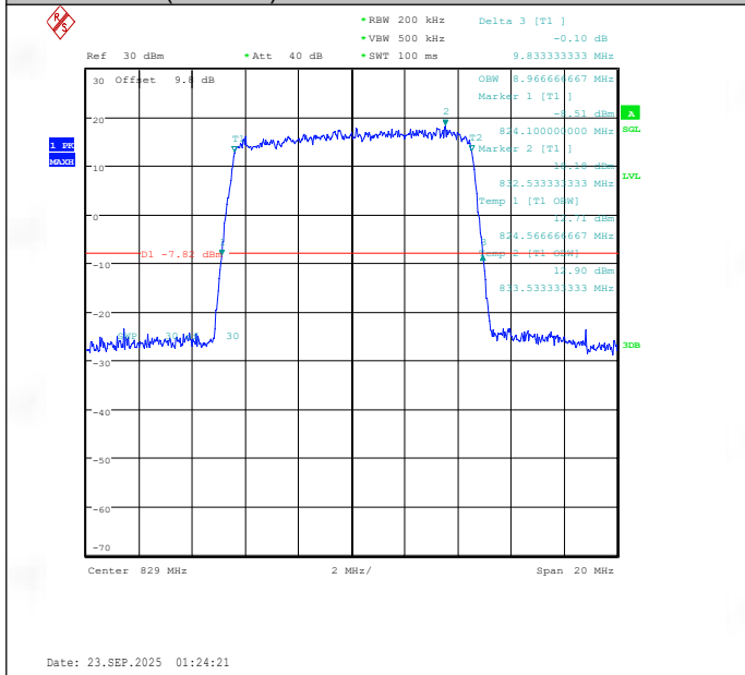
Band26(824-849)-10MHz-QPSK-26840-50RB#0-PASS
