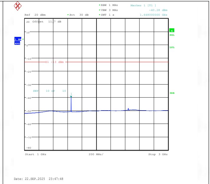
Band26(824-849)-3MHz-QPSK-26805-1RB#0-1000~3000-PASS
