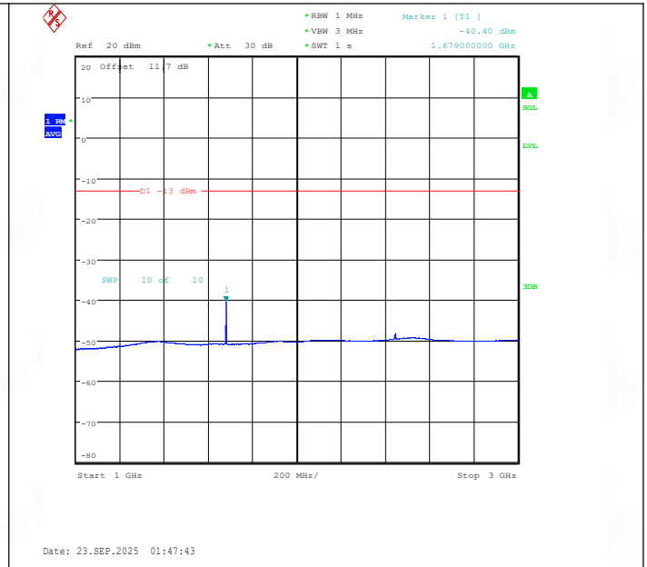
Band26(824-849)-10MHz-QPSK-26990-1RB#0-1000~3000-PASS
