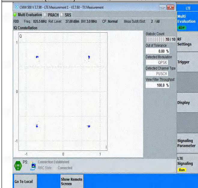
Band26(824-849)-3MHz-QPSK-26805-15RB#0-PASS
