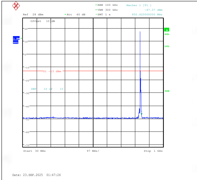
Band26(824-849)-10MHz-QPSK-26990-1RB#0-30~1000-PASS
