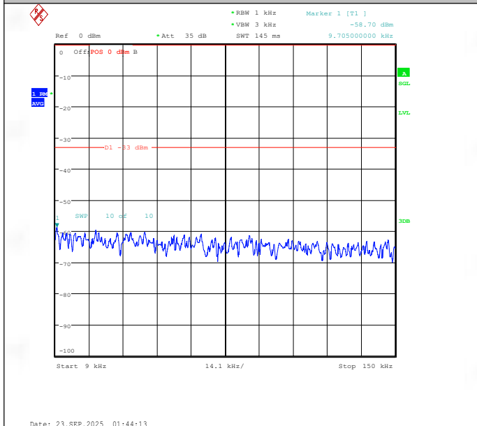
Band26(824-849)-10MHz-QPSK-26915-50RB#0-0.009~0.15-PASS
