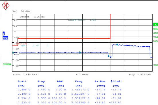
Band41(2535-2655)-20MHz-QPSK-40140-1RB#0-PASS
