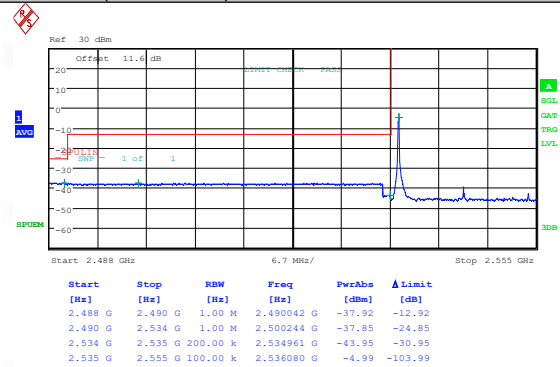
Band41(2535-2655)-20MHz-QPSK-40140-1RB#99-PASS
