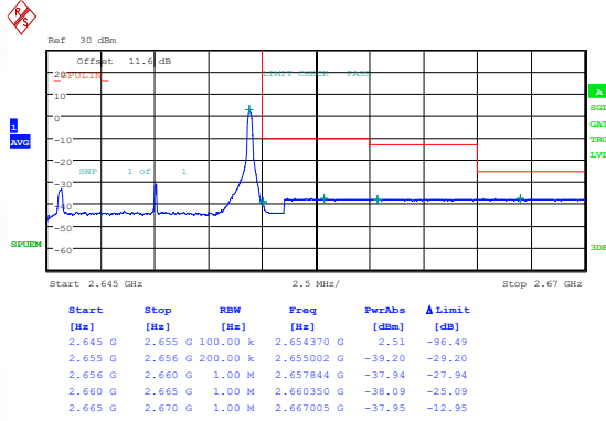
Band41(2535-2655)-10MHz-QPSK-41190-50RB#0-PASS
