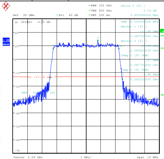
Band41(2535-2655)-5MHz-QPSK-40065-25RB#0-PASS
