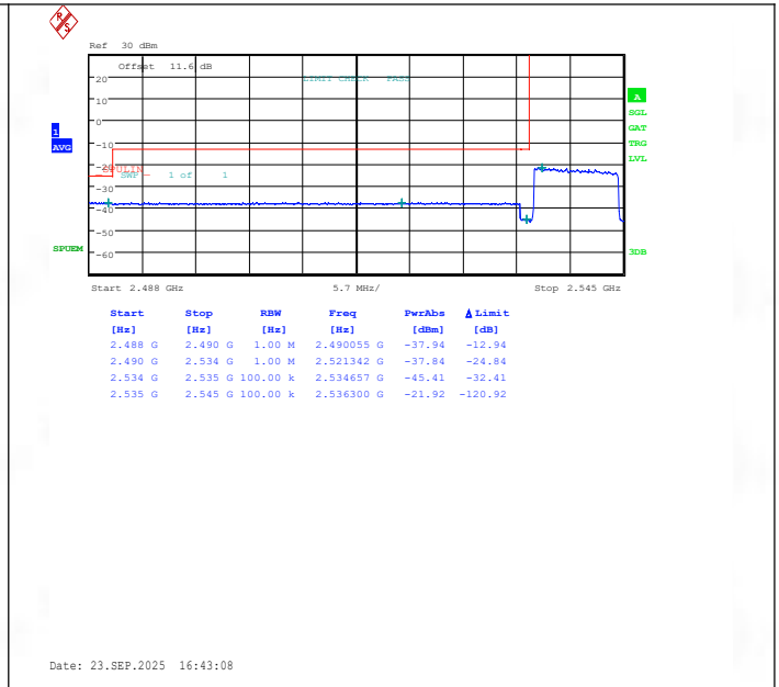
Band41(2535-2655)-10MHz-16QAM-40090-50RB#0-PASS
