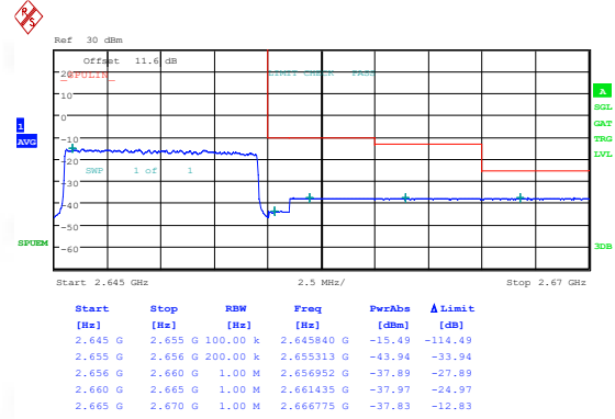
Band41(2535-2655)-10MHz-16QAM-41190-1RB#0-PASS
