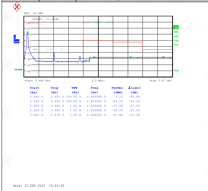
Band41(2535-2655)-10MHz-QPSK-41190-1RB#0-PASS
