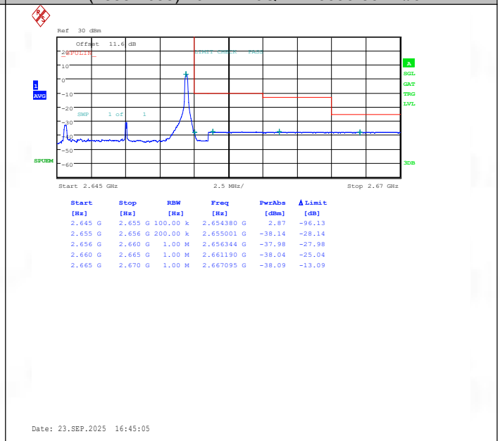
Band41(2535-2655)-10MHz-QPSK-41190-1RB#49-PASS
