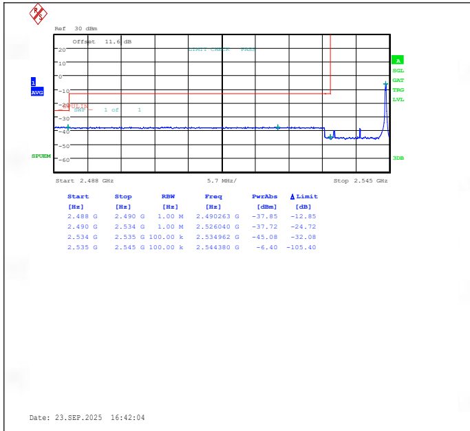
Band41(2535-2655)-10MHz-16QAM-40090-1RB#49-PASS
