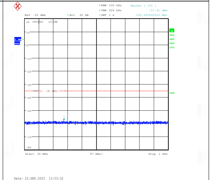
Band41(2535-2655)-20MHz-QPSK-40590-1RB#99-30~1000-PASS
