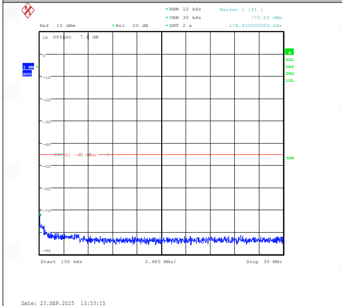
Band41(2535-2655)-20MHz-QPSK-40590-1RB#99-0.15~30-PASS
