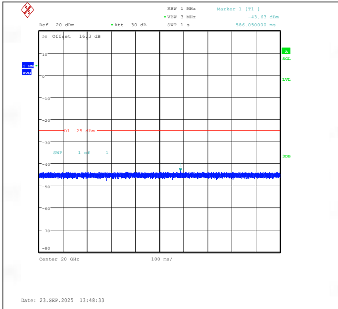
Band41(2535-2655)-20MHz-QPSK-40590-1RB#0-20000~27000-PASS
