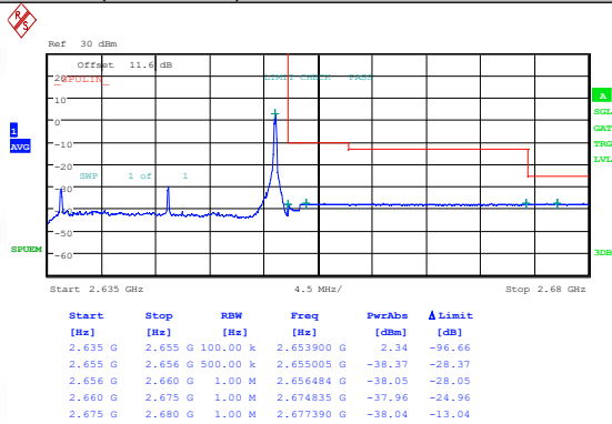
Band41(2535-2655)-20MHz-QPSK-41140-100RB#0-PASS
