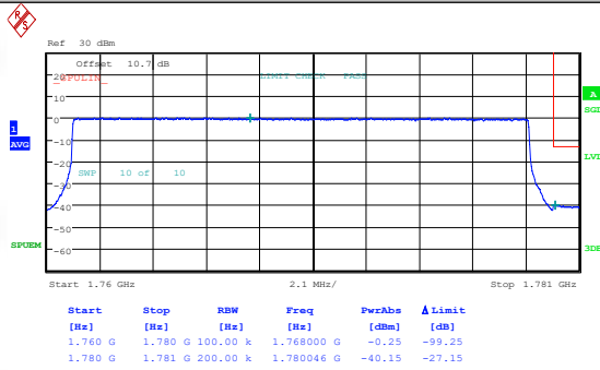
Band66-20MHz-QPSK-132572-1RB#0-PASS
