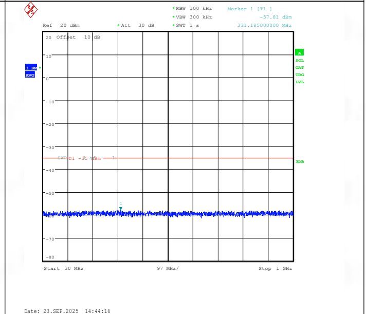
Band41(2535-2655)-10MHz-QPSK-40590-1RB#49-30~1000-PASS
