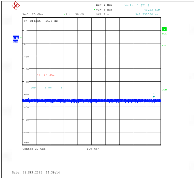
Band41(2535-2655)-10MHz-QPSK-40590-1RB#0-20000~27000-PASS
