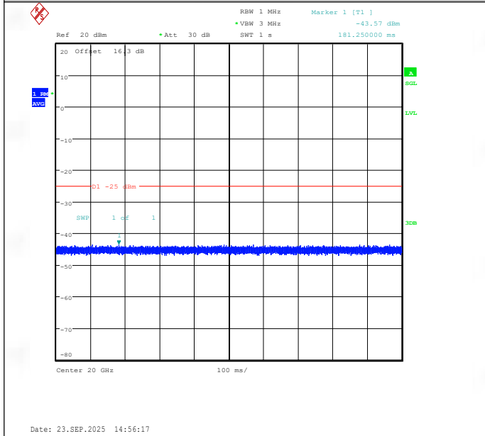
Band41(2535-2655)-10MHz-QPSK-41190-1RB#0-20000~27000-PASS
