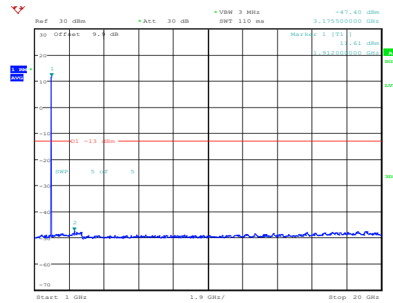
Band25-1.4MHz-QPSK-26683-1RB#0-Range4:1000~20000MHz
