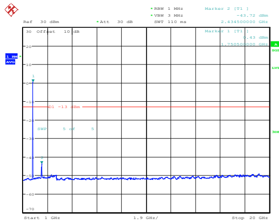
Band4-1.4MHz-QPSK-20393-1RB#0-Range4:1000~20000MHz
