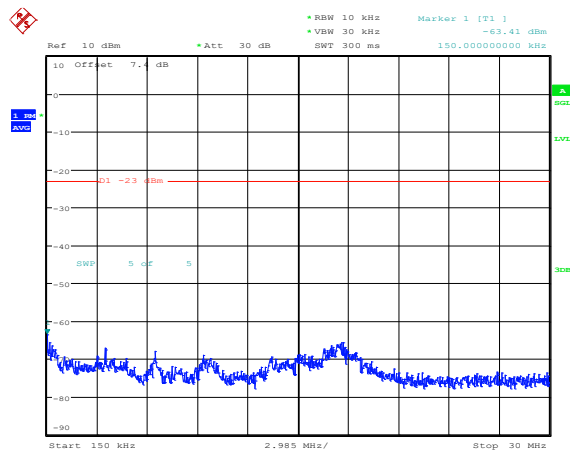
Band4-5MHz-QPSK-19975-1RB#0-Range2:0.15~30MHz
