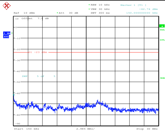
Band4-1.4MHz-QPSK-19957-1RB#0-Range2:0.15~30MHz
