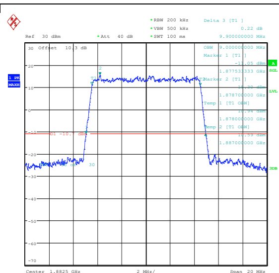
Band25-10MHz-16QAM-26365-50RB#0-PASS
