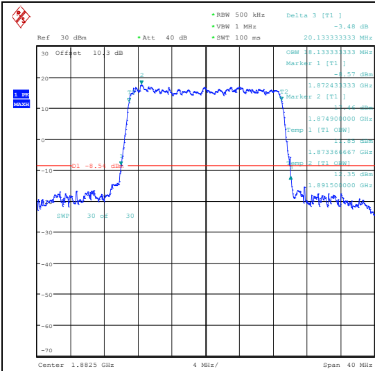
Band25-20MHz-QPSK-26365-100RB#0-PASS
