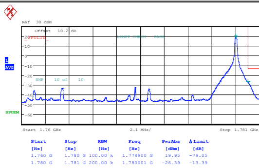
Band66_20MHz_QPSK_132572_1RB#0
