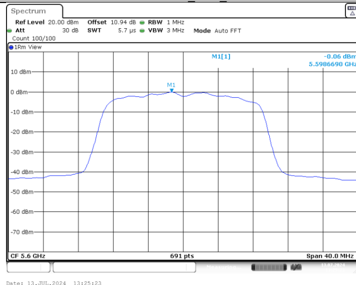
11AC20MIMO_Ant2_5600
