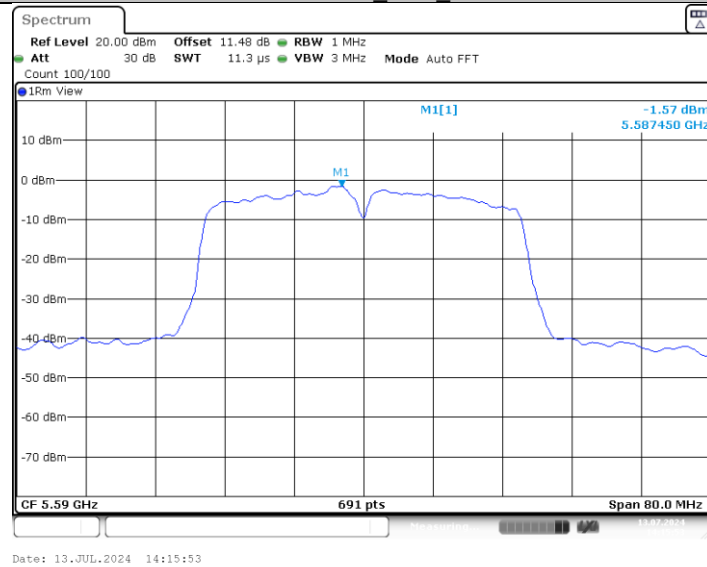
11AC40MIMO_Ant2_5590
