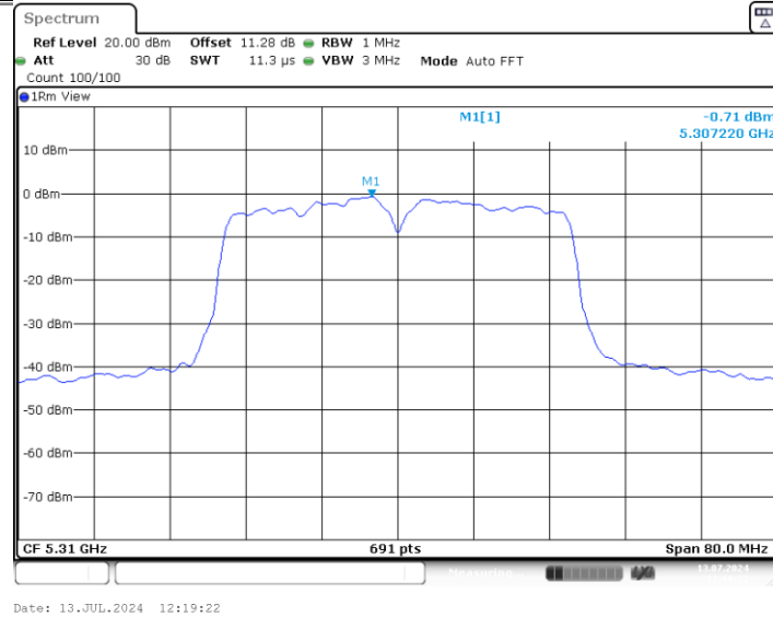
11N40MIMO_Ant2_5310
