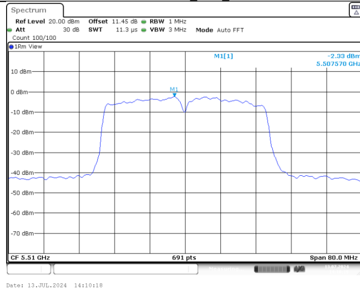
11AC40MIMO_Ant2_5510
