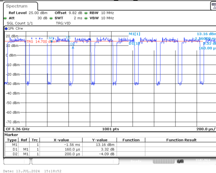
11AX20MIMO_Ant2_5260
