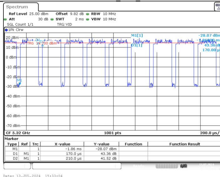
11AX20MIMO_Ant2_5320
