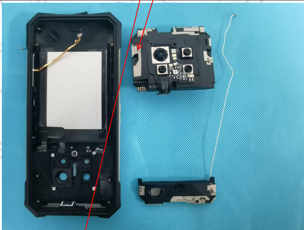
GPS&amp;BT&amp;WiFi 2.4G/5G_ANT
