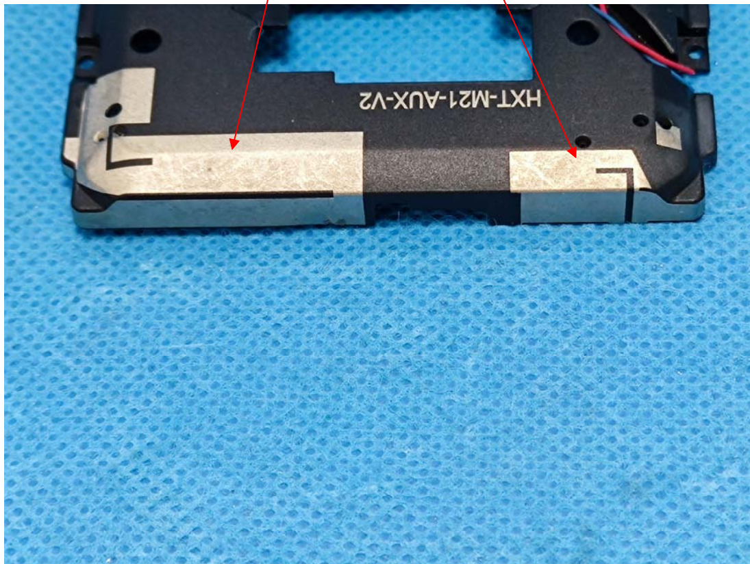
Bluetooth/WiFi Antenna WWAN Aux Antenna
