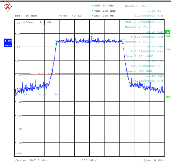
Band26(824-849)-3MHz-16QAM-26915-15RB#0-P ASS
