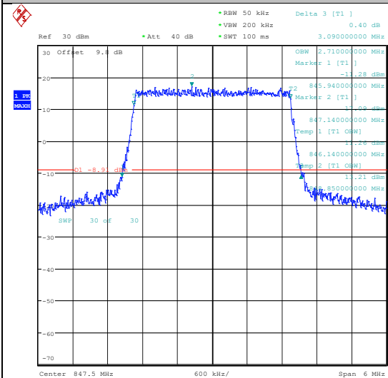
Band26(824-849)-3MHz-QPSK-26915-15RB#0-P ASS
