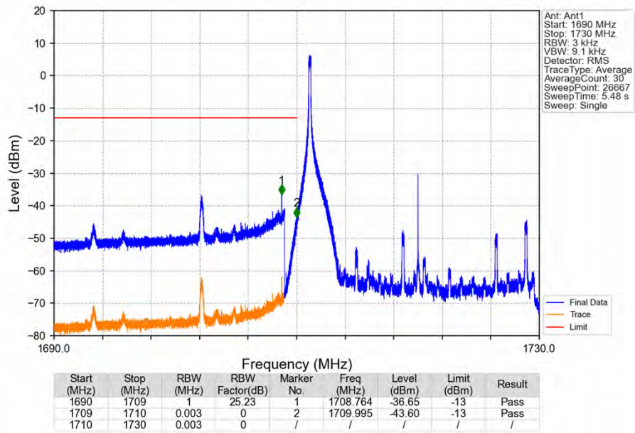
Band66_20MHz_16QAM_LCH_1720MHz_RB_1_0_NTNV
