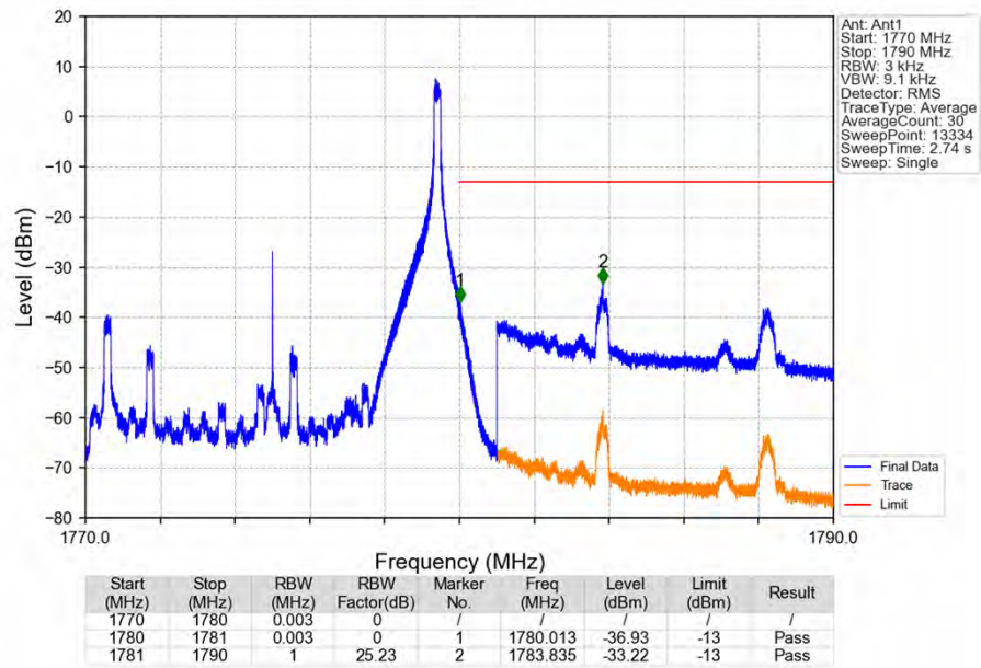
Band66_10MHz_QPSK_HCH_1775MHz_RB_1_49_NTNV
