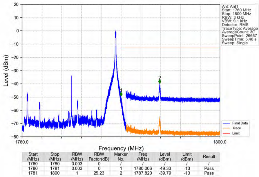
Band66_20MHz_16QAM_HCH_1770MHz_RB_1_99_NTNV
