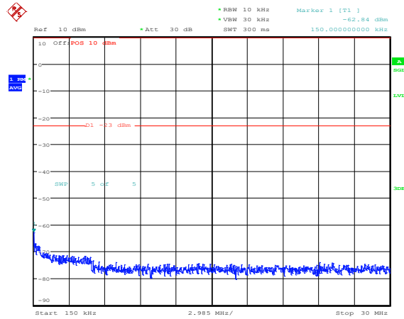
Band25-5MHz-QPSK-26365-1RB#0-Range2:0.15~30MHz
