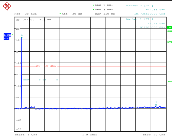
Band25-1.4MHz-QPSK-26683-1RB#0-Range4:1000~20000MHz
