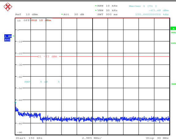
Band25-3MHz-QPSK-26055-1RB#0-Range2:0.15~30MHz
