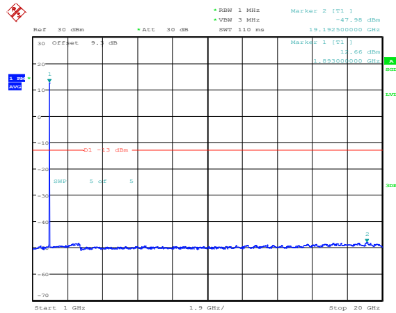
Band25-15MHz-QPSK-26615-1RB#0-Range4:1000~20000MHz
