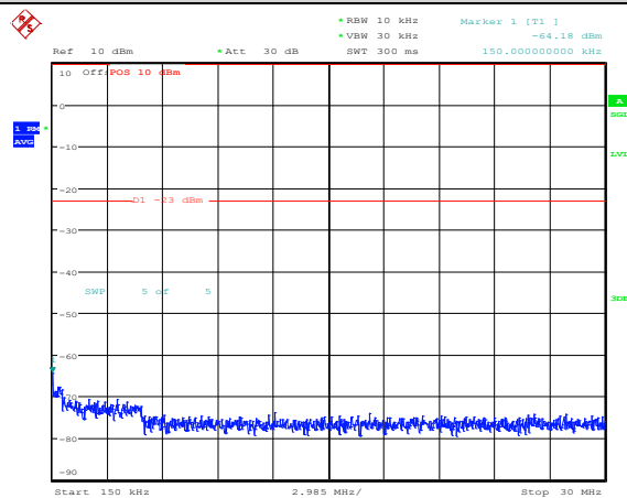
Band25-3MHz-16QAM-26365-1RB#0-Range2:0.15~30MHz
