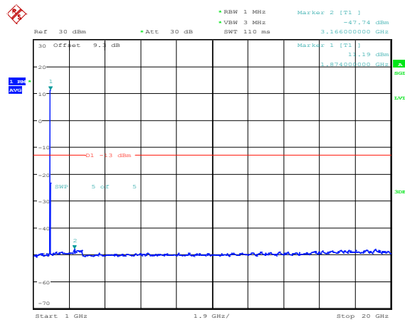
Band25-10MHz-QPSK-26365-1RB#0-Range4:1000~20000MHz
