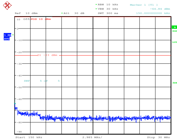
Band25-10MHz-QPSK-26365-1RB#0-Range2:0.15~30MHz
