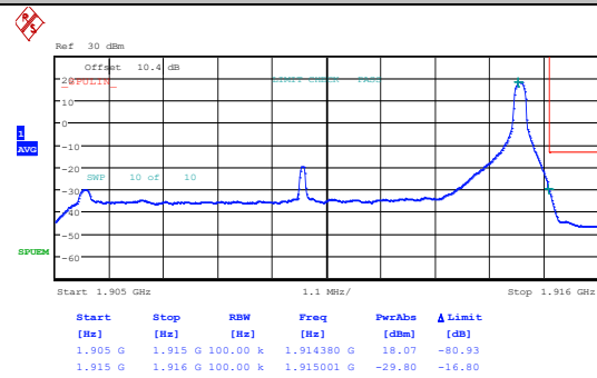
Band25-10MHz-QPSK-26640-50RB#0-PASS
